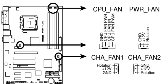
P5B-PLUS Fan connectors
