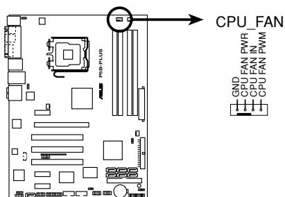
P5B-PLUS CPU fan connector
