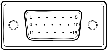
图八 15 针彩色显示器信号线
