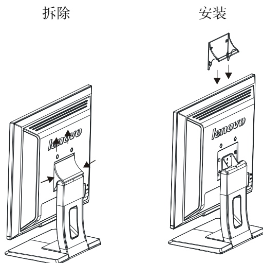
图二 拆除和安装转轴盖
