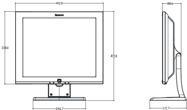
图七 外观尺寸
