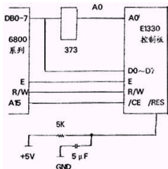
6800 的连接
