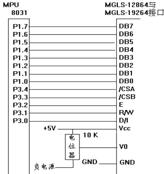
图八 间接控制方式原理图
