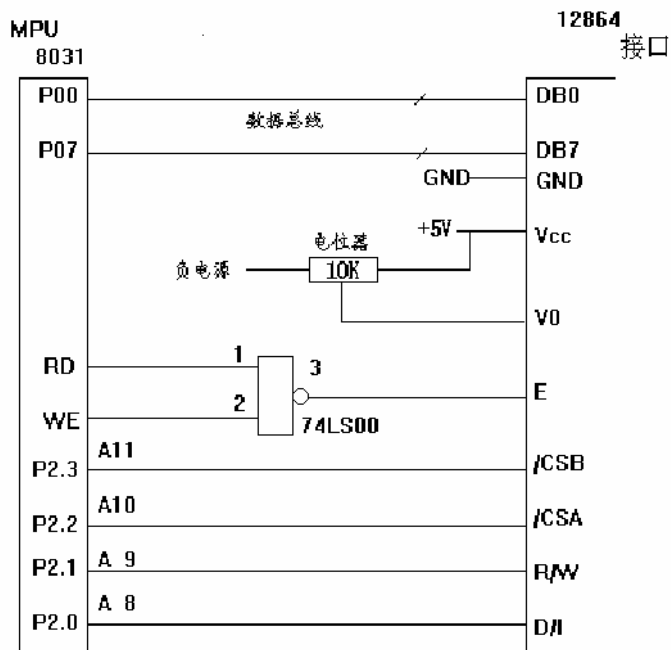
图七 直接访问方式原理图
