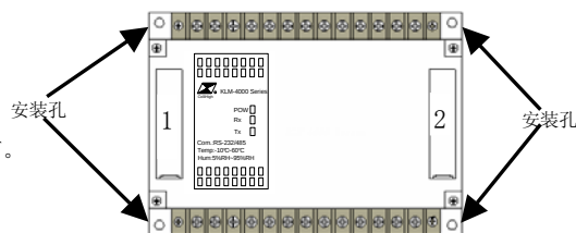
图 2-3 安装示意图
