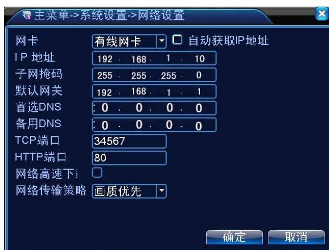
图 4.17 网络设置
