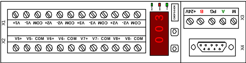
（图 1）CMDF5-8ADK 端子示意图
