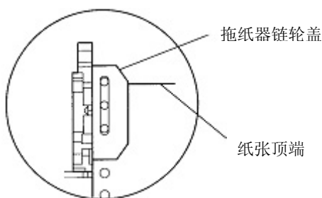
图 3-9 安装连续纸于拖纸器齿轮上
