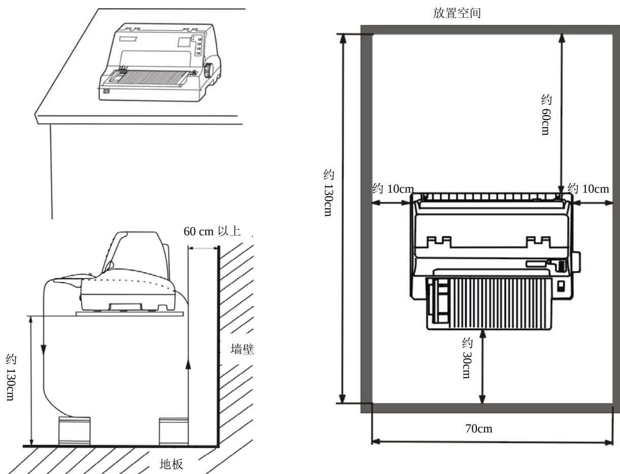
图 2-5 打印机放置
