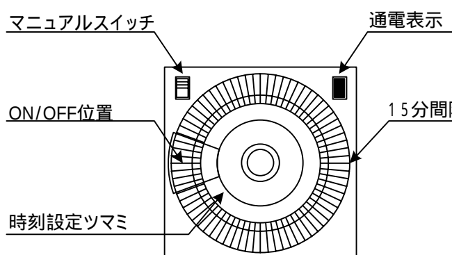
タイマー取付外形図
