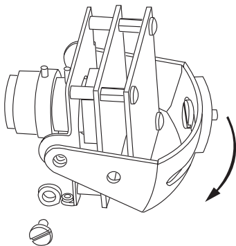
图3 调整摄像机角度
