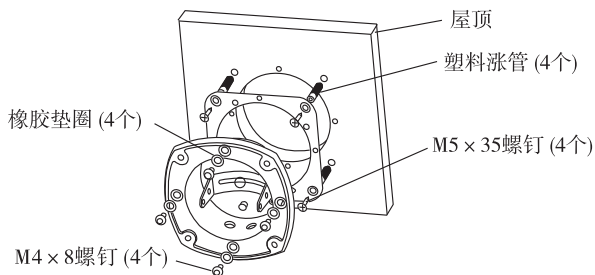
图6 暗装云台安装
