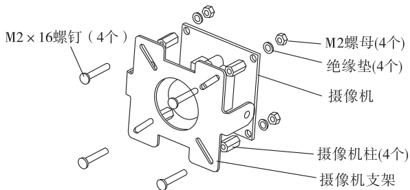
图1 固定镜头
