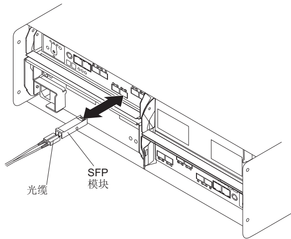
图 85. 更换 SFP 模块
