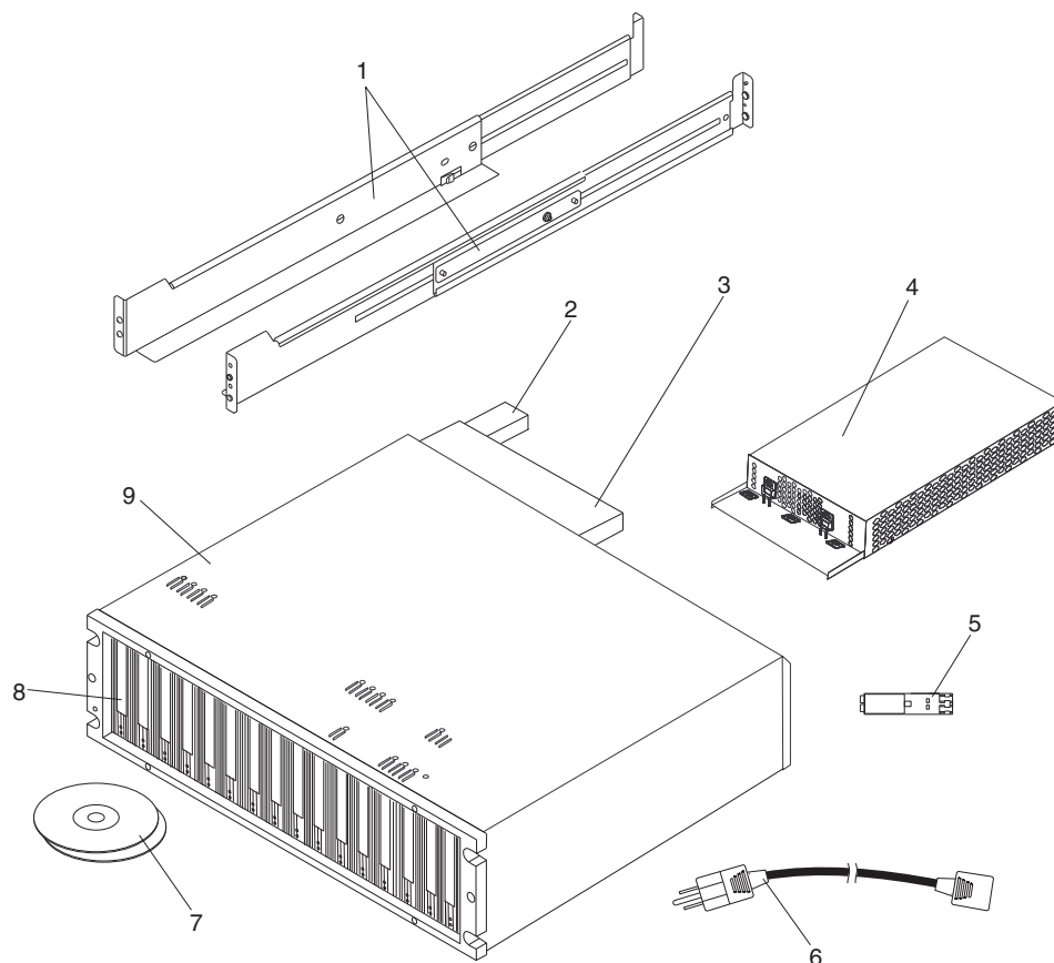
图 88. DS5020 存储子系统部件列表
