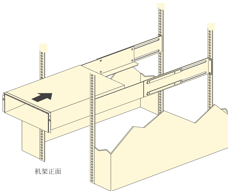
图 19. 安装 DS5020
