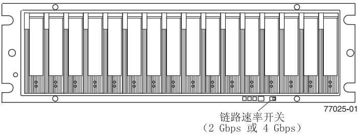
图 82. “链路速率”开关
