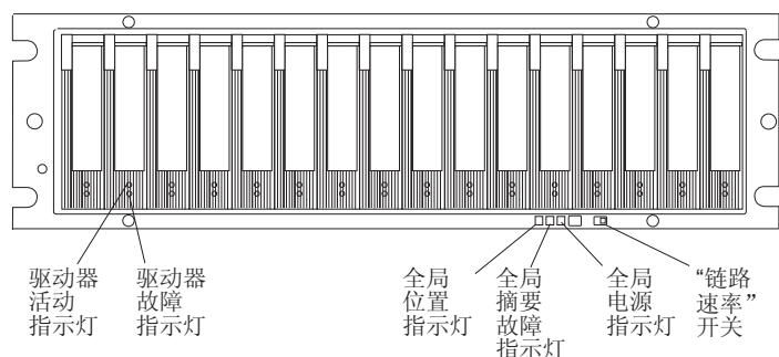
图 67. 前部指示灯和控制件
