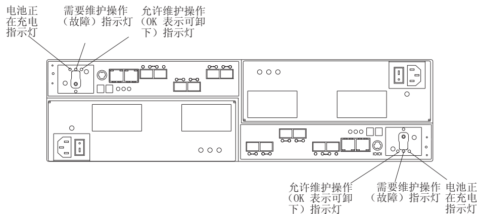
图 68. 电池单元指示灯
