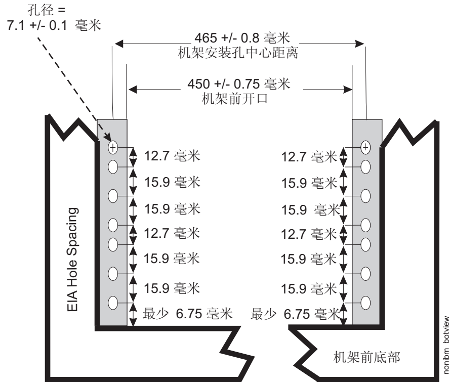
图 93. 机架规格尺寸，底视图（前部）
