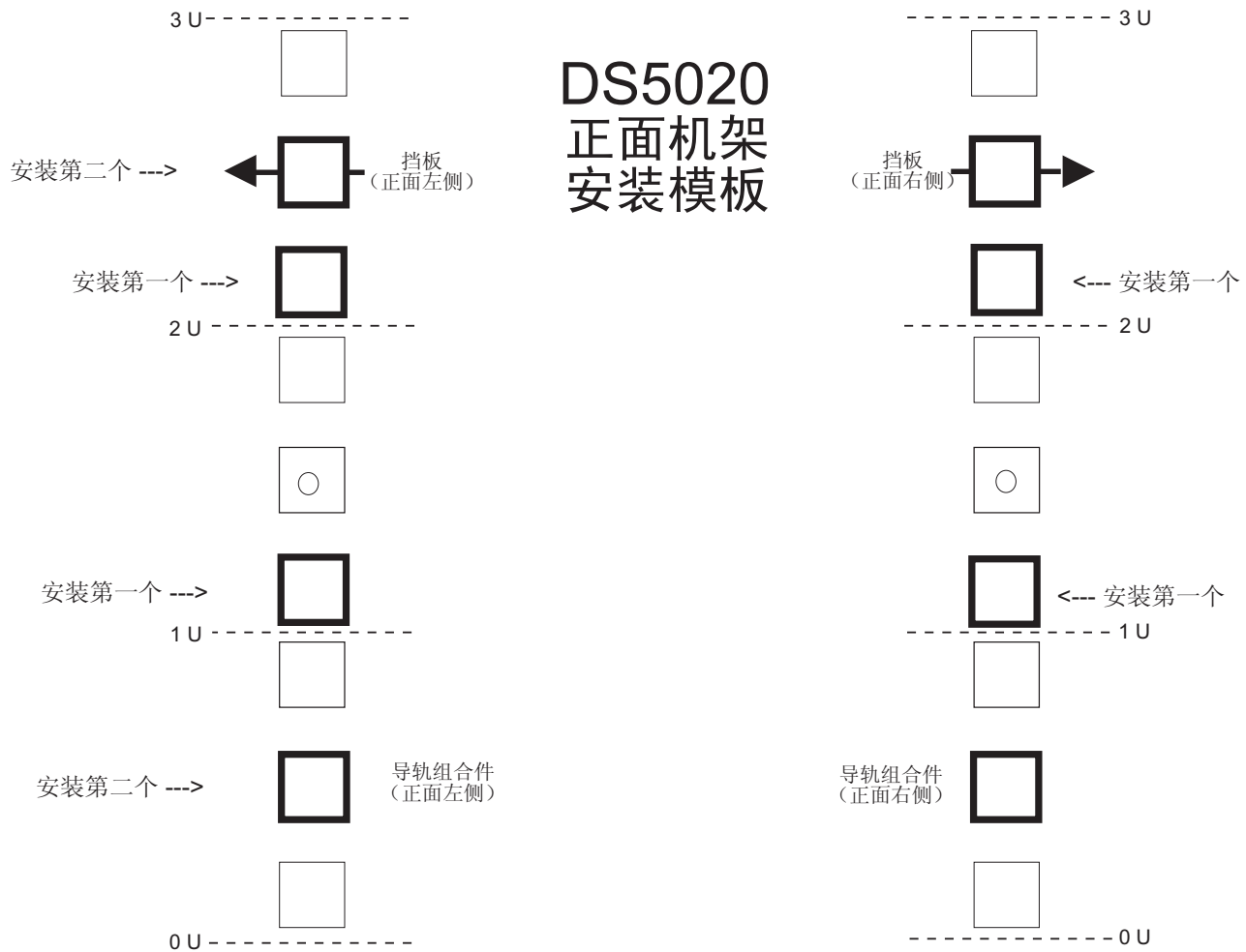
图 89. 前部机架安装模板
