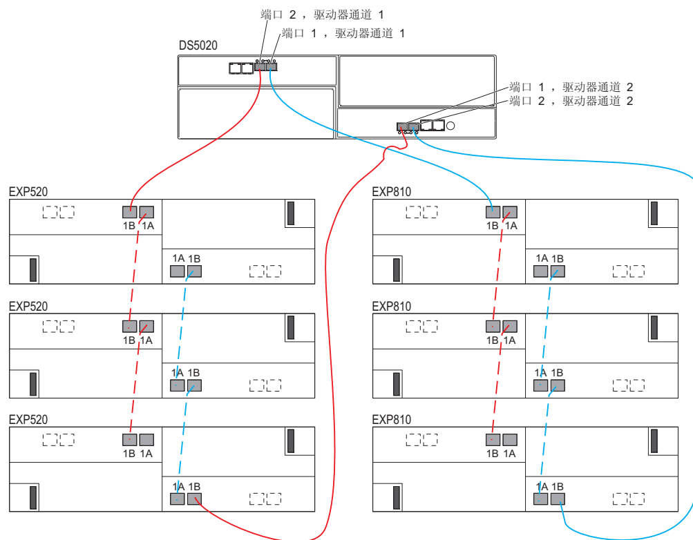
图 44. 用电缆连接混合环境中的一个 DS5020 和两个或更多个存储扩展机柜
