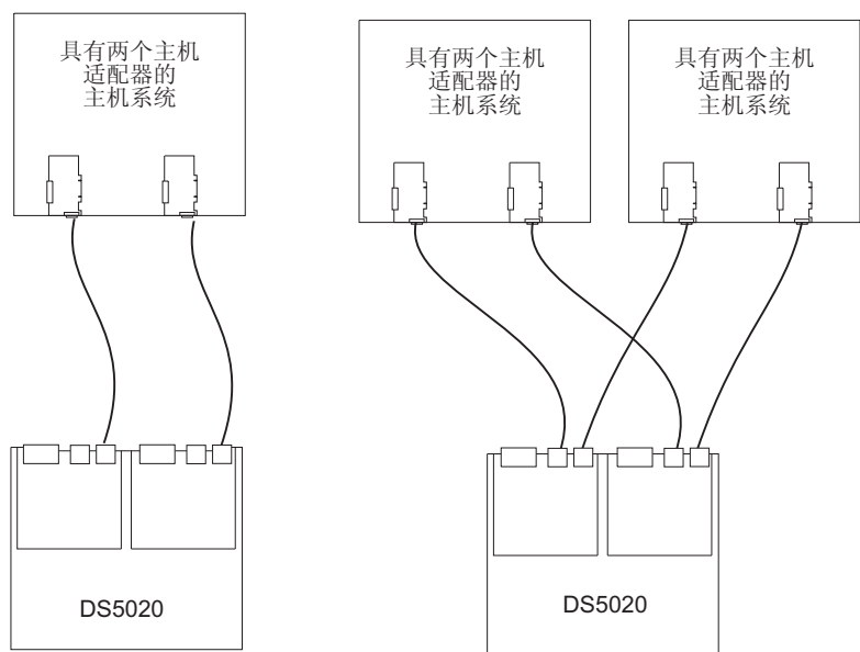
图 56. 冗余主机直接连接光纤通道 SAN 配置示例
