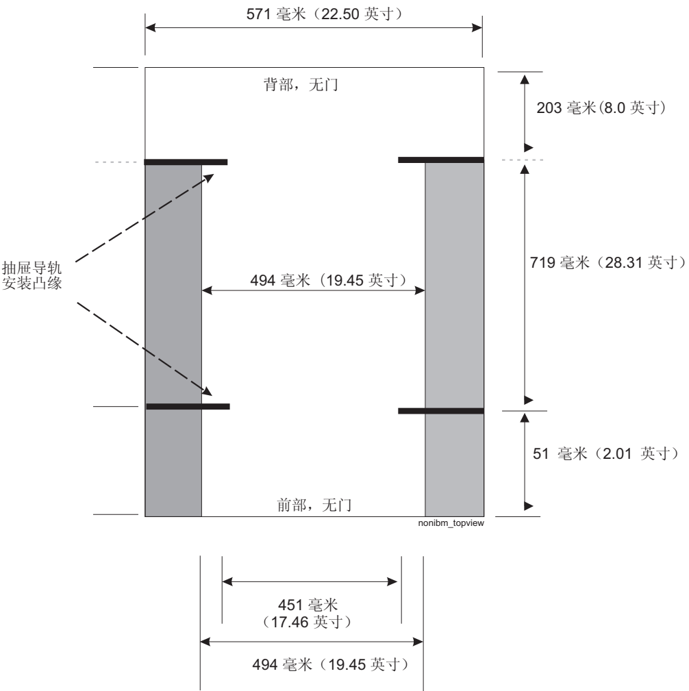
图 91. 非 IBM 机架规格尺寸的顶视图
