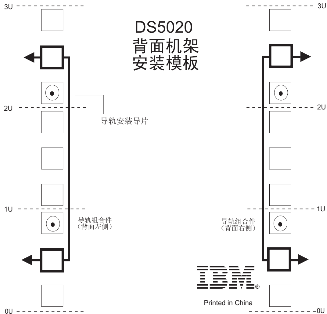
图 90. 后部机架安装模板
