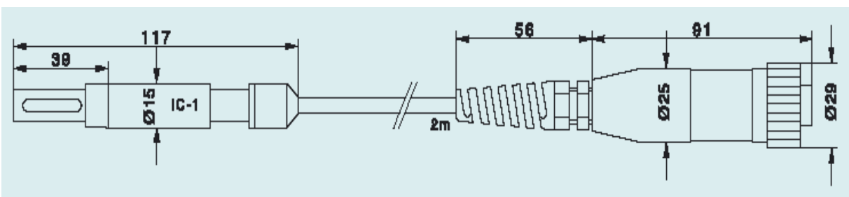
外形尺寸图:
