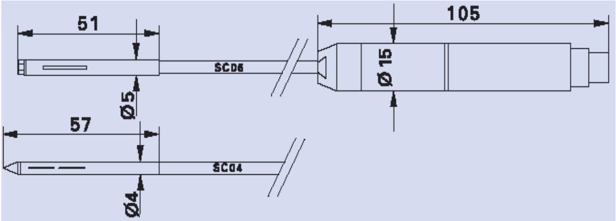
外形尺寸图：
