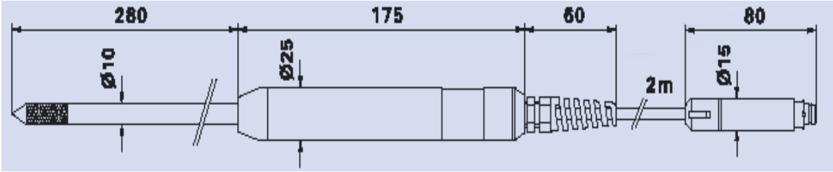
外形尺寸图:
