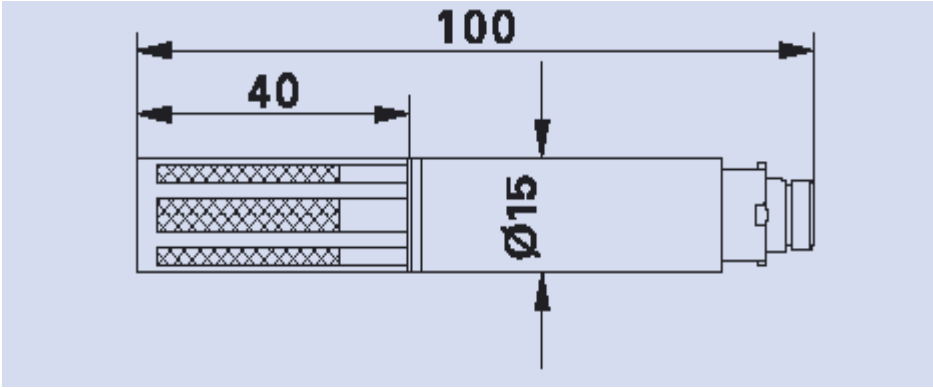
外形尺寸图：
