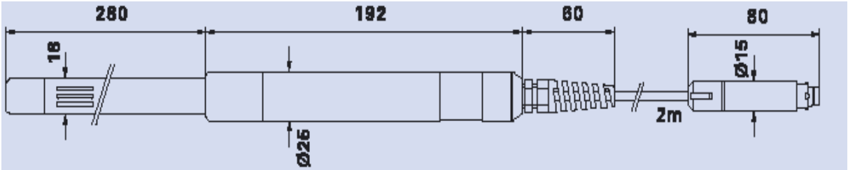
外形尺寸图:
