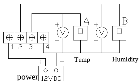
0-5V output
