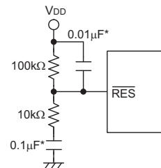
复位电路
