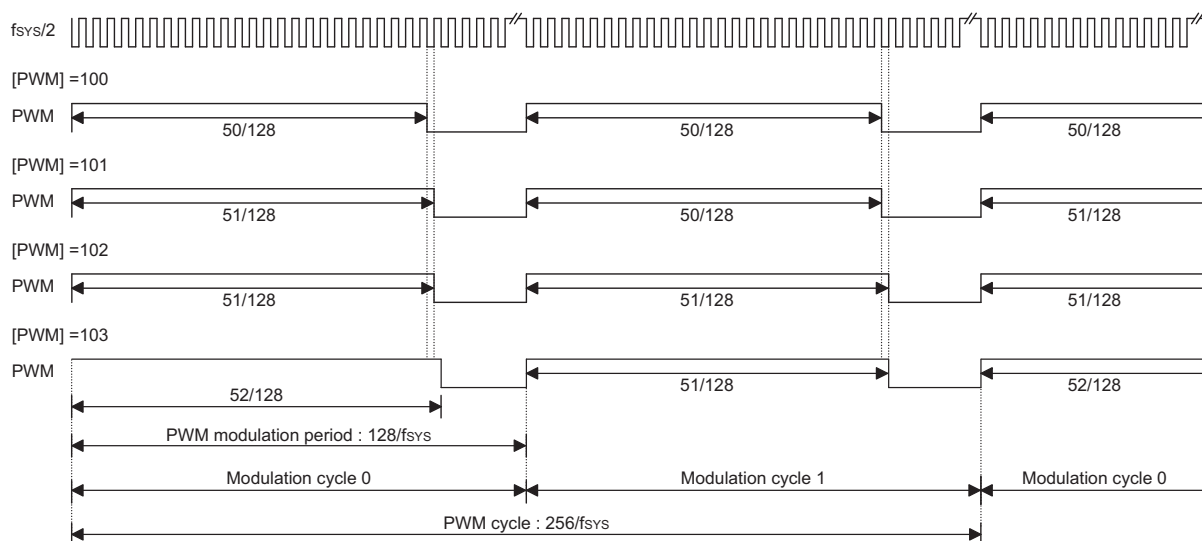
(7+1)位模式 PWM
