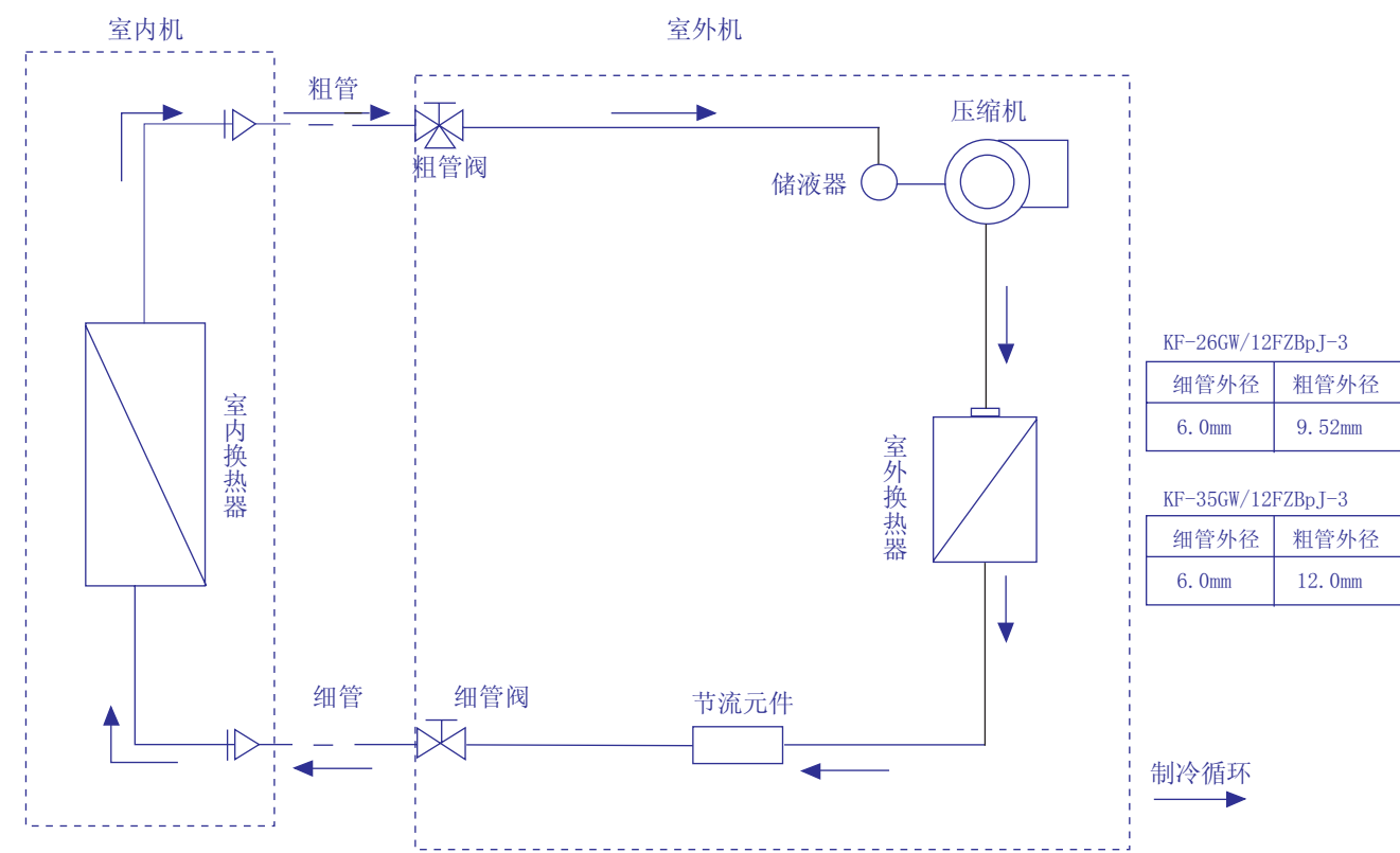
制冷剂循环流程图
