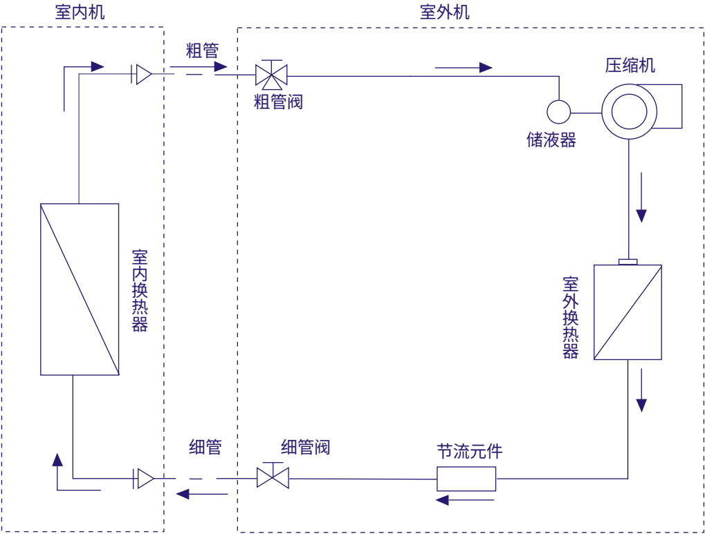
制冷剂循环流程图
