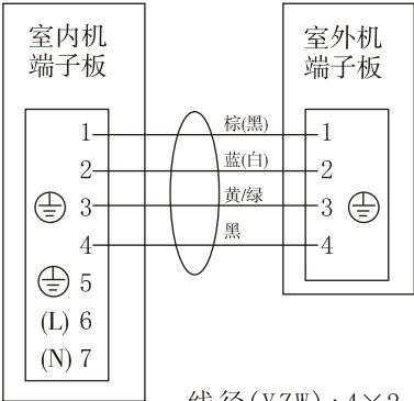
线径(YZW)：4×2.5mm²
