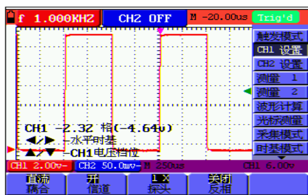
图 36: 直流耦合
