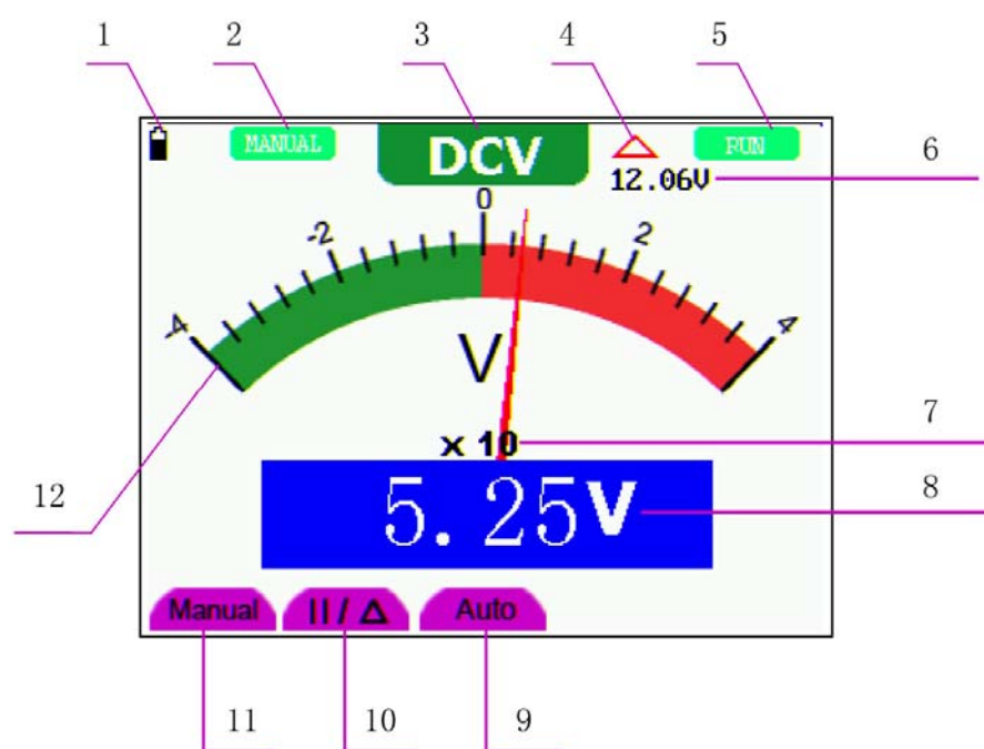
图 20：万用表界面
