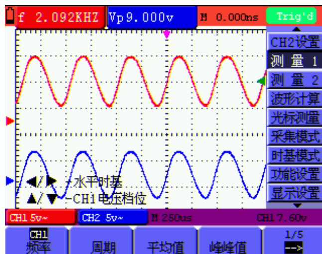
图 12：自动测量
