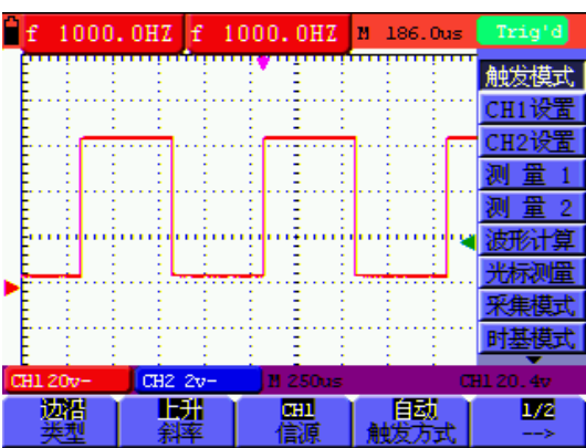
图40 边沿触发（第一页）
