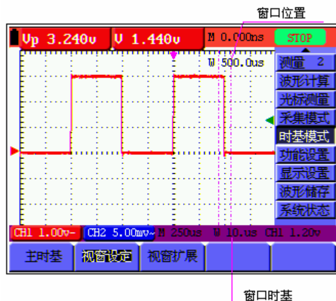
图58：视窗设定
