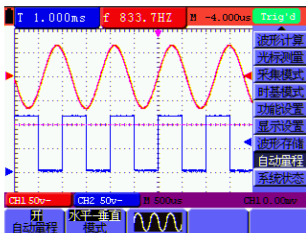
图 53 自动量程 水平---垂直模式多周期波形图
