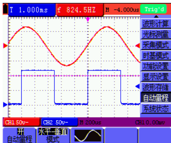
图 54 自动量程 水平---垂直模式单周期波形图
