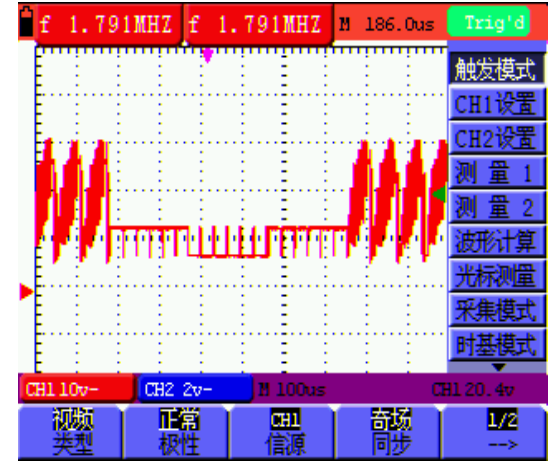
图42 视频奇场触发（第一页）
