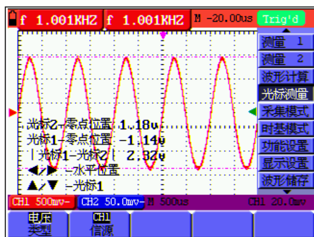
图 51: 光标电压测量
