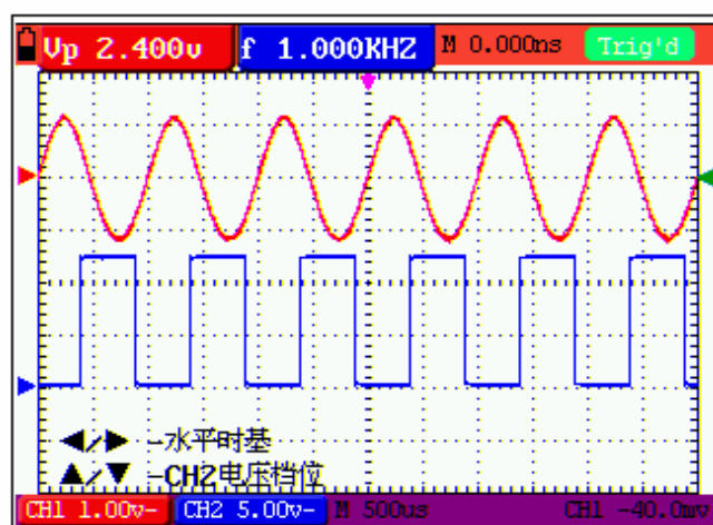
图 7: CH2 电压档位显示界面
