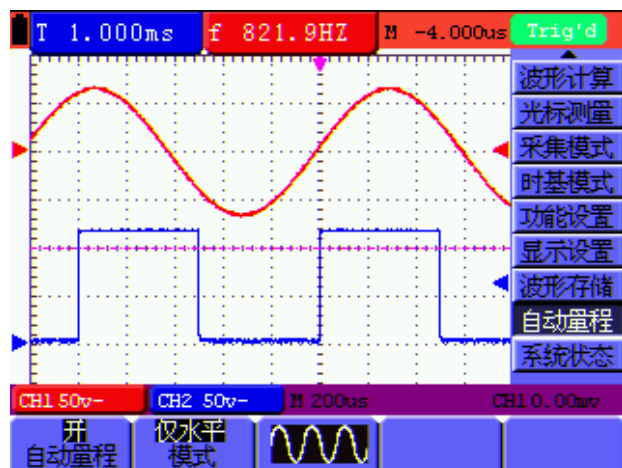
图 56 仅水平模式多周期
