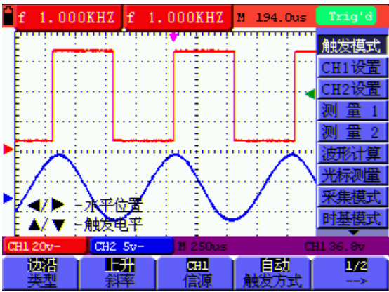
图 39：边沿触发
