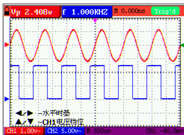
图 6: CH1 电压档位显示界面
