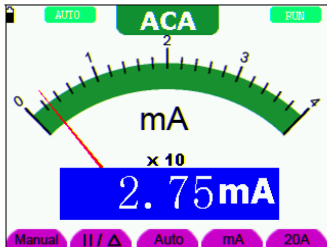
图 29: 交流电流测量界面
