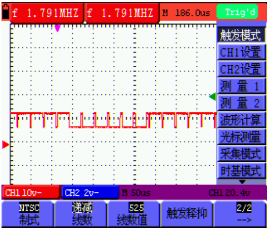
图45 视频指定行触发（第二页）
