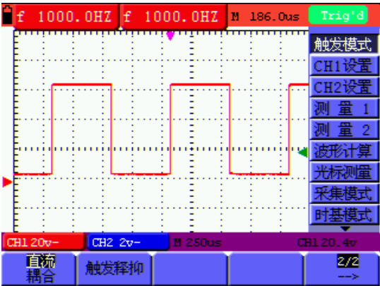
图41 边沿触发（第二页）
