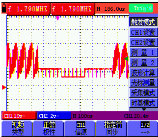
图44 视频指定行触发（第一页）
