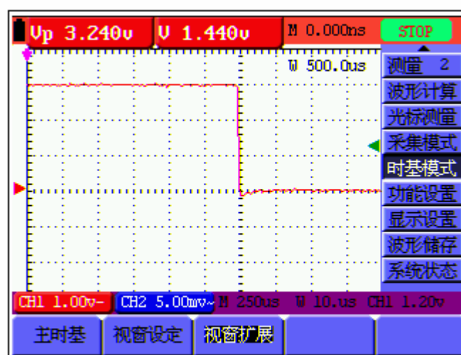
图59：视窗扩展
