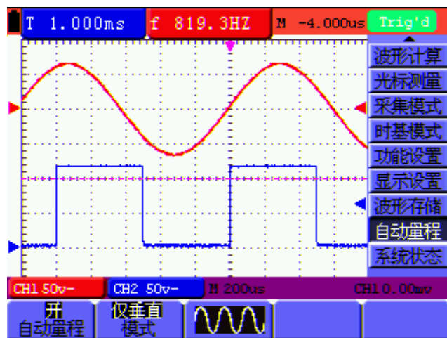
图 55 自动量程仅垂直模式多周期
