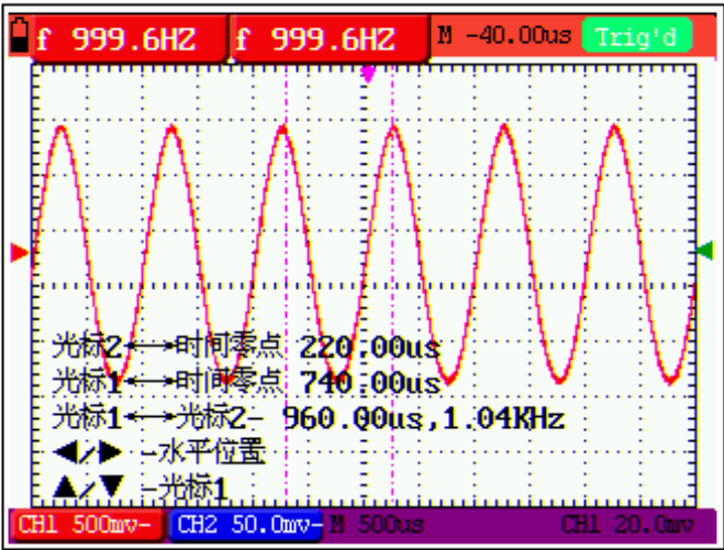
图 52：光标时间测量
