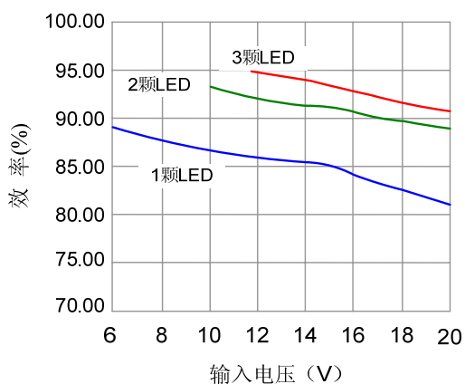
输出 350mA 效率随输入电压变化曲线
