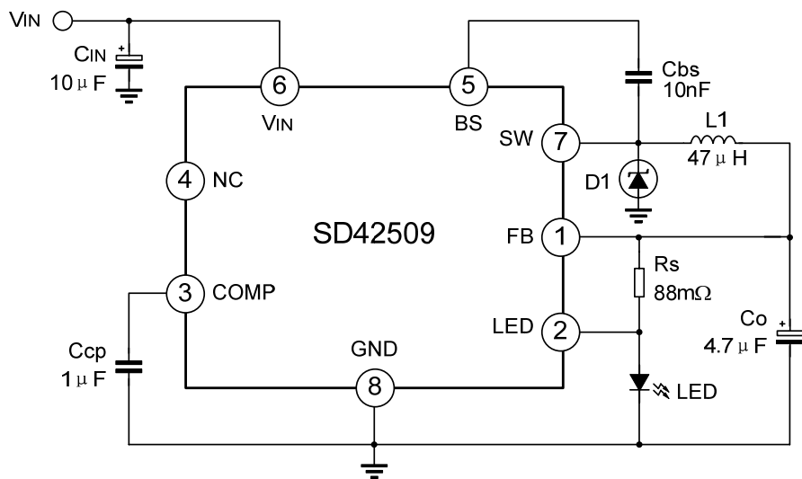
6~20V 输入电压，1A 输出 LED 驱动电路
