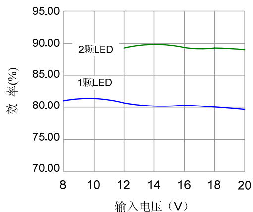
输出 1A 效率随输入电压变化曲线
