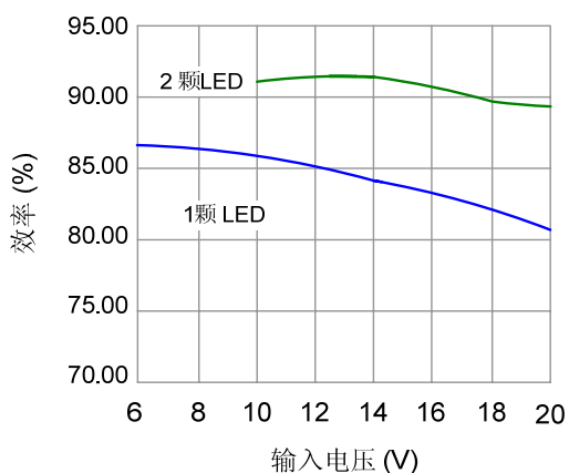
输出 700mA 效率随输入电压变化曲线
