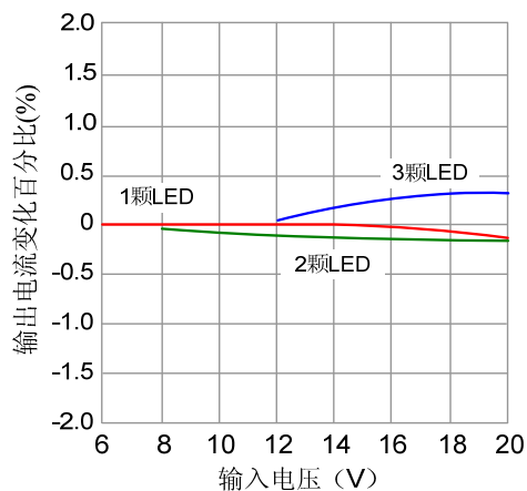
输出 700mA 电流随输入电压变化率
