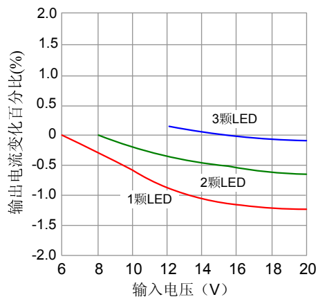
输出 350mA 电流随输入电压变化率
