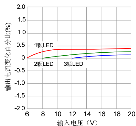
输出 1A 电流随输入电压变化率
