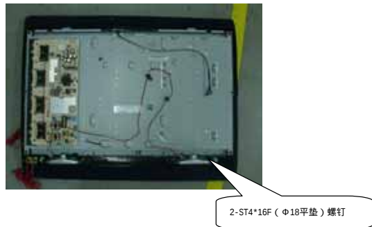
3. 整机拆卸之-----喇叭的拆卸
