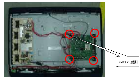
4. 整机拆卸之-----机芯板的拆卸
