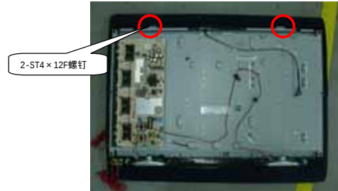
2. 整机拆卸之-----压片的拆卸
