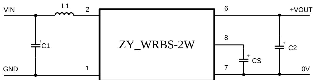
图 4.1 ZY_WRBS-2W 接口电路
