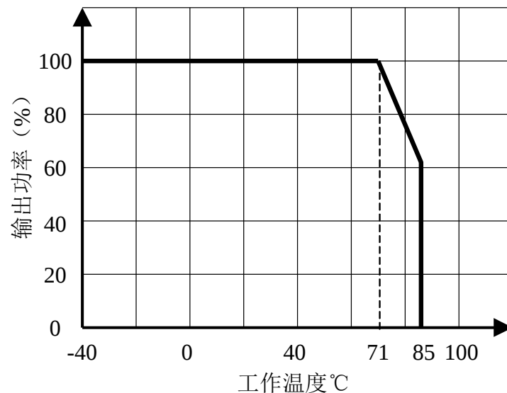
图 2.2 工作温度与输出功率曲线图
