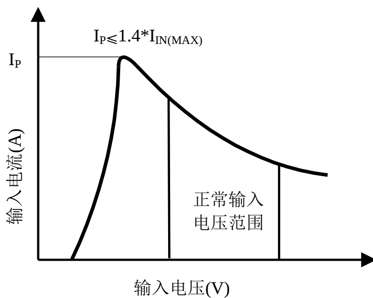
图 2.3 输入电流与输入电压曲线图
