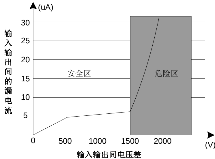
图 2.1 绝缘特性曲线图
