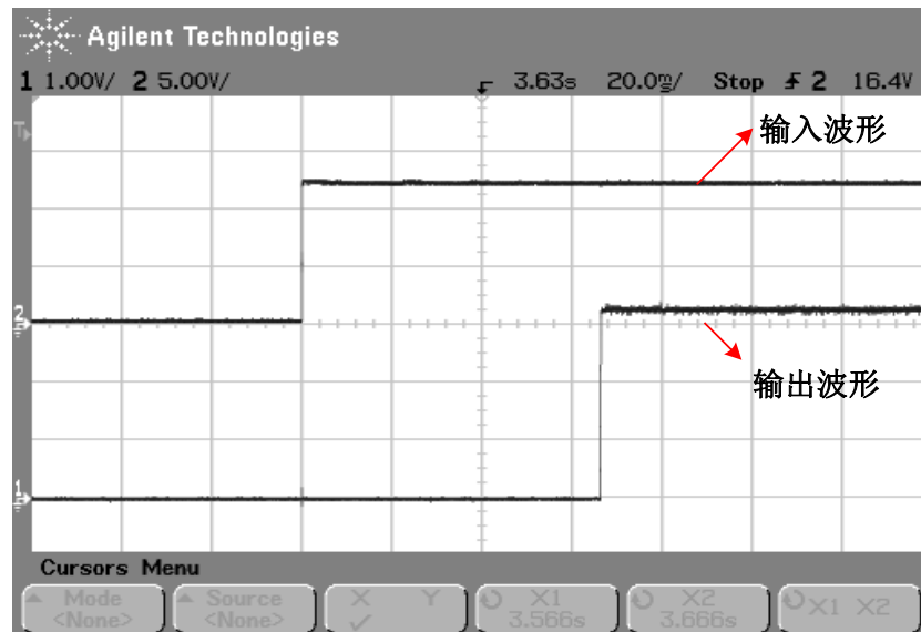
图 2.5 启动波形
