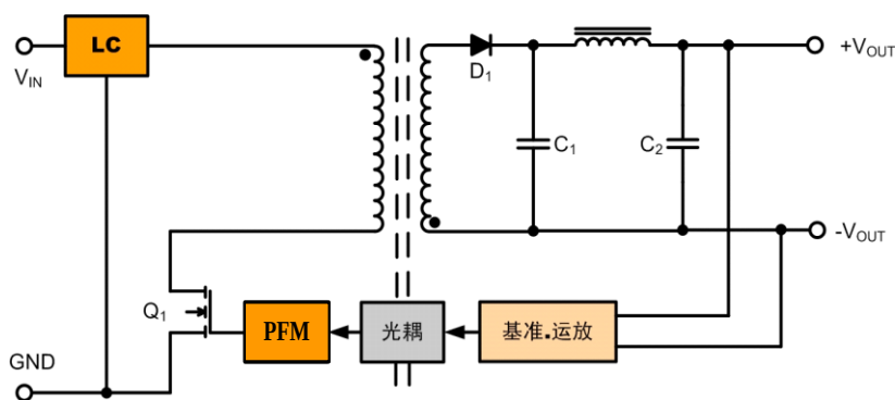
图 1 原理框图
