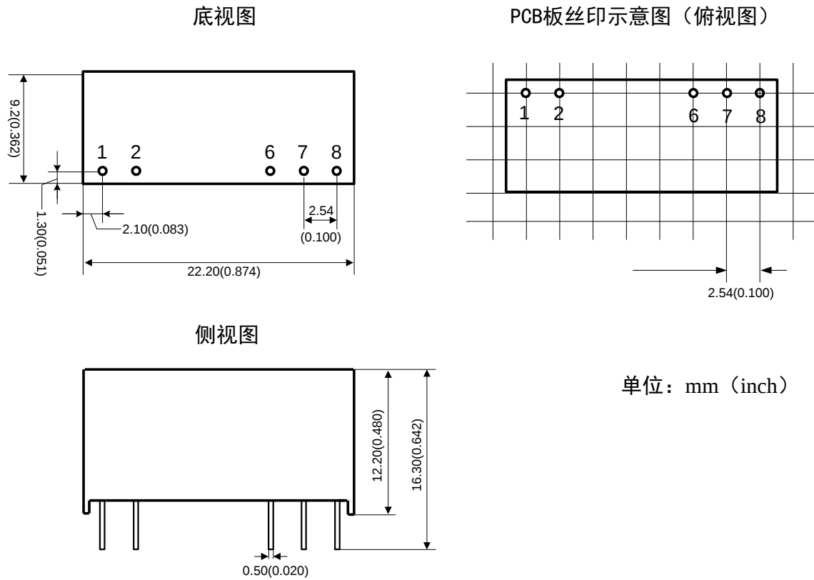
图 6.1 ZY_WRBS-2W 机械尺寸图
