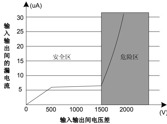
图 2.1 绝缘特性曲线图
