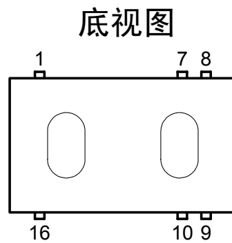
图 4.2 ZY_WRBD-2W 引脚封装图
