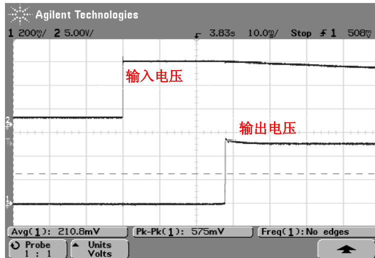
图 2.4 启动波形
