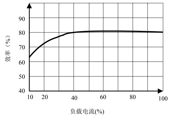
效率VS 负载电流
