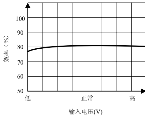
效率VS输入电压
