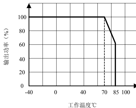
图 2.2 工作温度与输出功率曲线图
