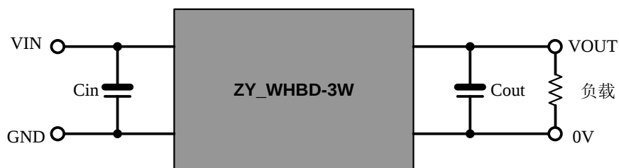
图 5.1 ZY_WHBD-3W 电源模块工作电路连接
