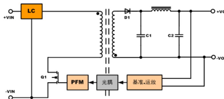
图 1 原理框图
