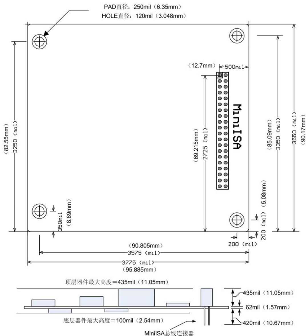
图 2.2 EPC-2901 工控主板机械尺寸
