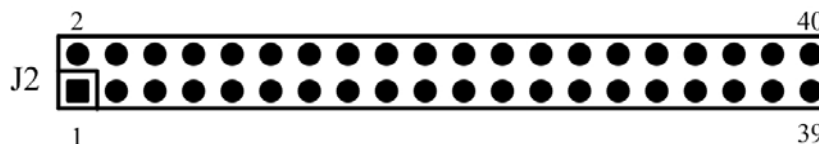
图 2.7 MiniISA 接口
