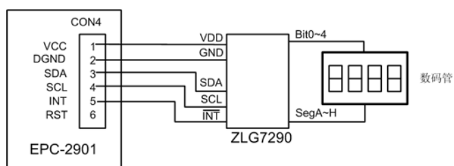
图 2.28 ZLG7290 驱动 LED 电路连接图
