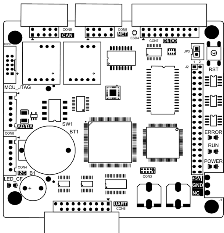
图 2.1 EPC-2901 工控主板硬件结构图
