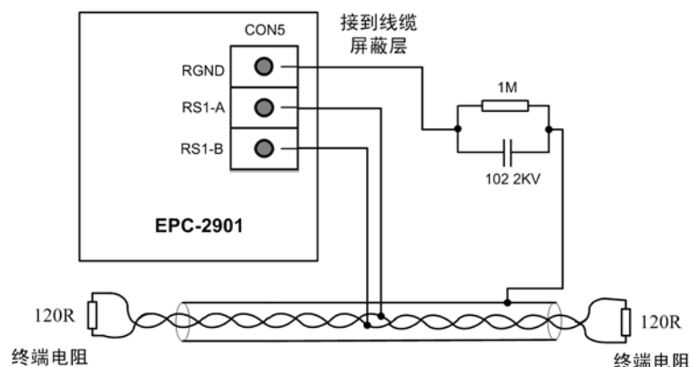
图 2.21 CAN 总线屏蔽层连接示意图
