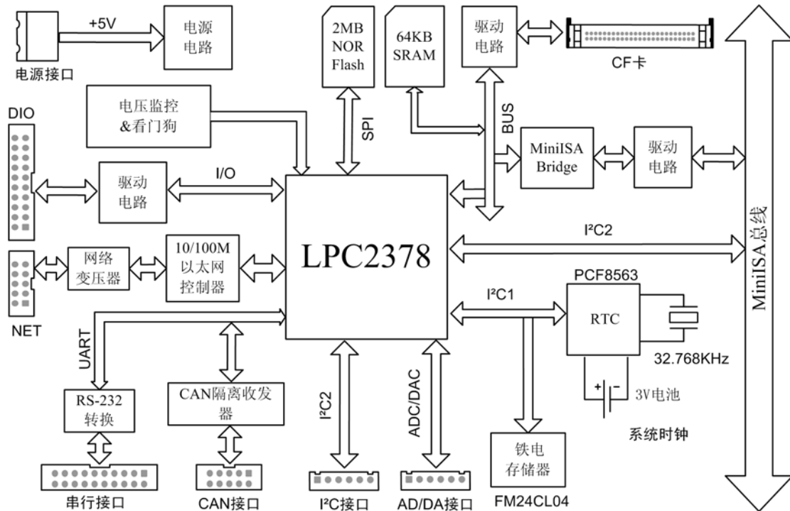
图 1.2 EPC-2901 工控主板系统结构框图
