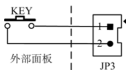
图 2.10 外部复位连接示意图
