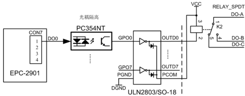
图 2.17 GPO 光耦隔离输出电路示意图
