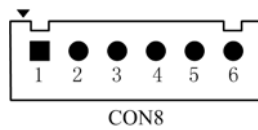
图 2.18 A/D、D/A 接口管脚排列
