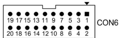
图 2.24 4 路 RS-232C 接口
