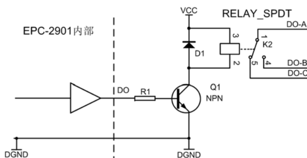
图 2.16 继电器输出示意图
