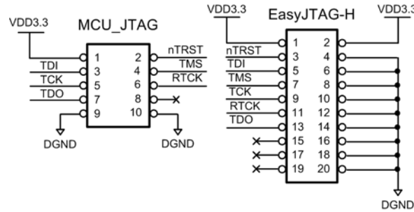
图 2.12 10 针 JTAG 接口与 20 针 H-JTAG 的接线图
