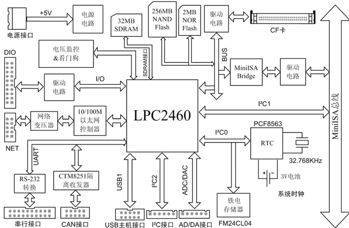
图 2.1 EPC-3100 工控主板系统结构框图
