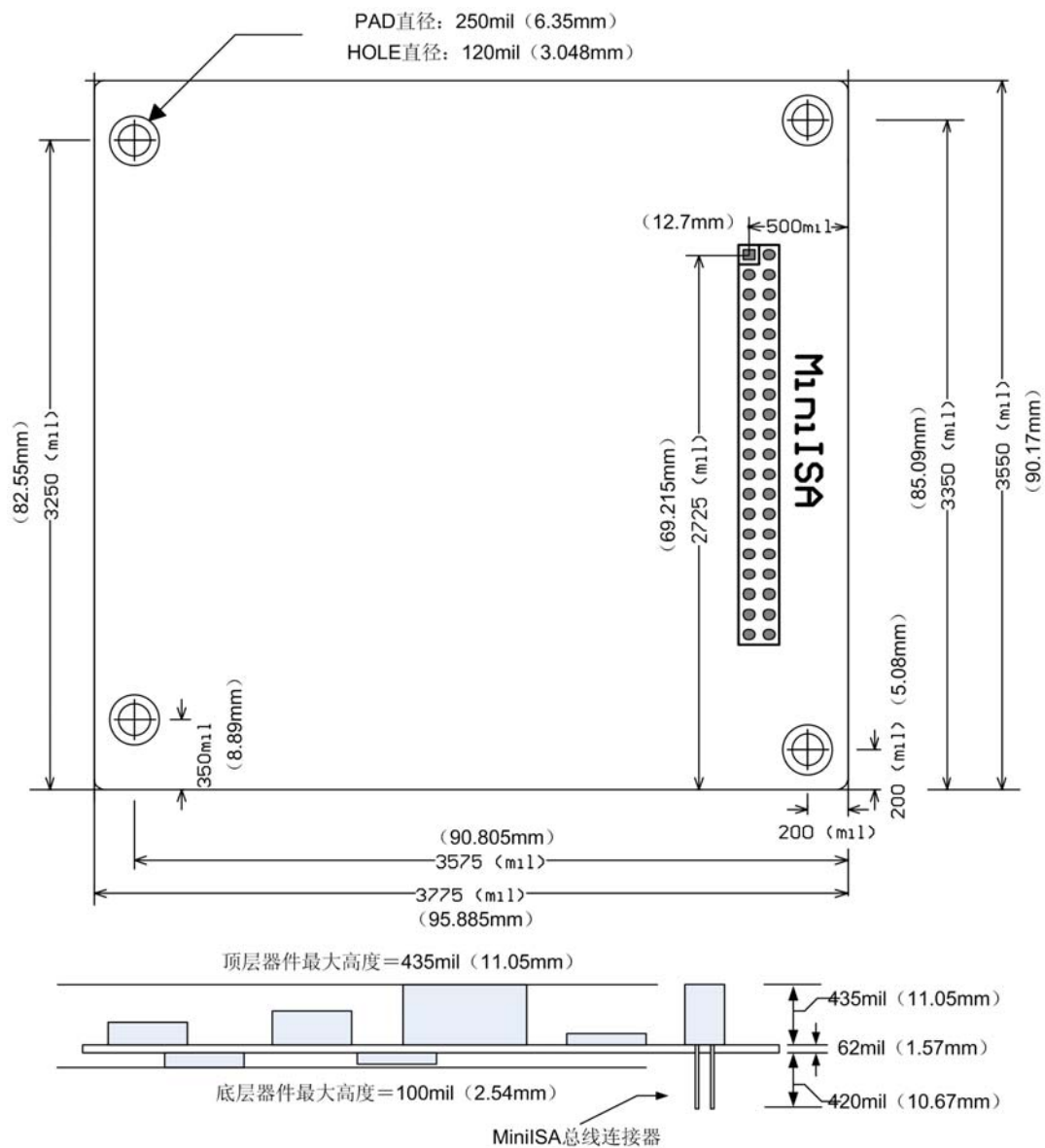
图 4.1 EPC-3100 工控主板机械尺寸
