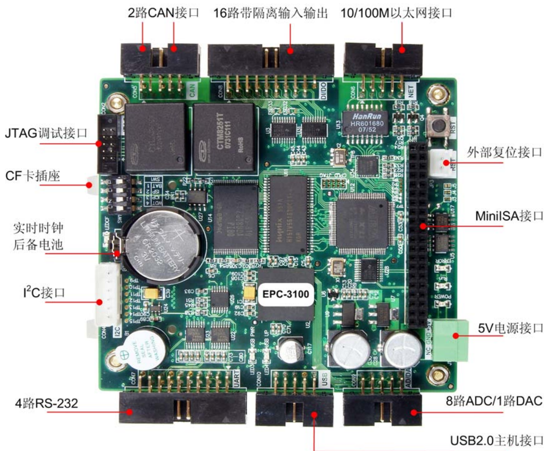
图 1.2 EPC-3100 实物图
