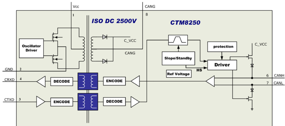
图 1.1 CTM8250 芯片功能框图
