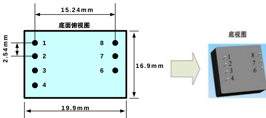
图 2.2 CTM8250 引脚封装
