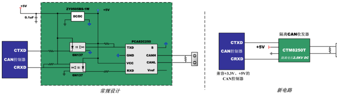
图 1 CTM8250 应用示例
