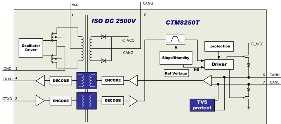
图 1.2 CTM8250T 芯片功能框图
