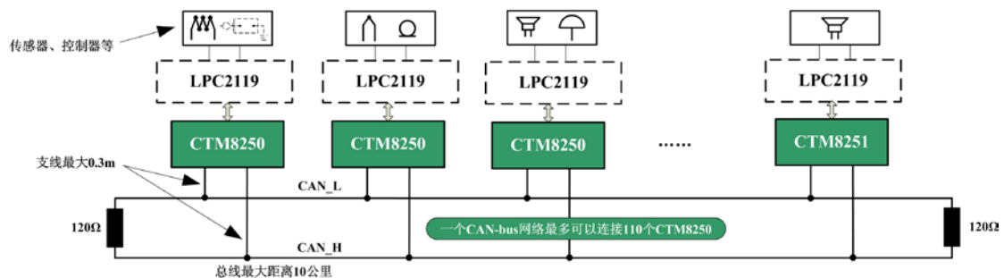
图 5.2 CTM8250 典型应用
