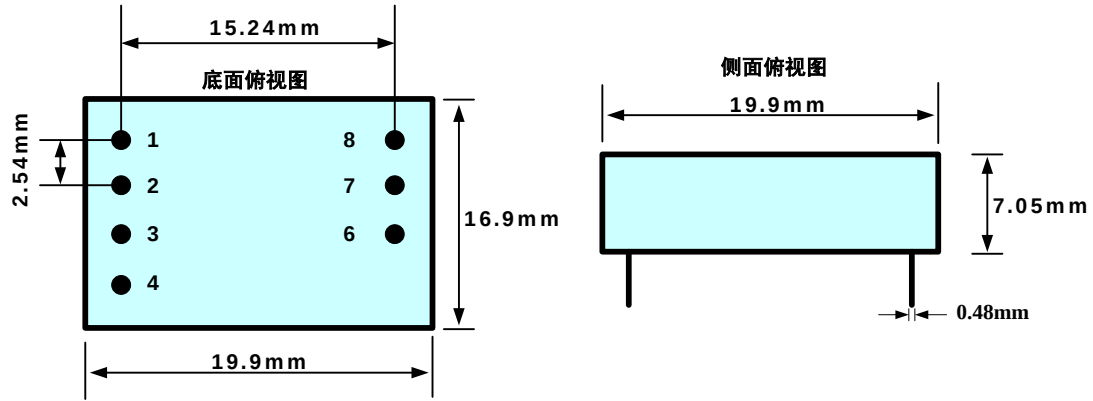
图 4.1 CTM8250 外观机械尺寸
