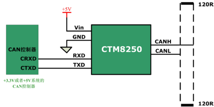
图 5.1 CTM8250 接口电路
