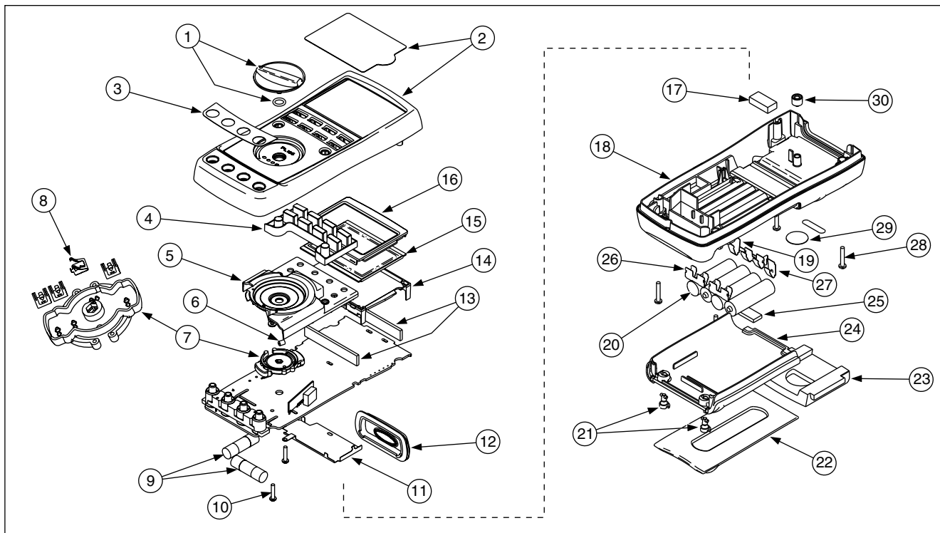
圖 12. 更換零件
