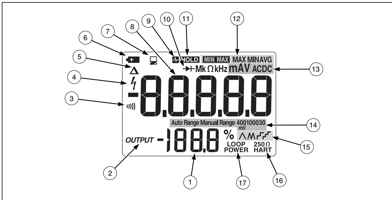
图 6. 显示单元
