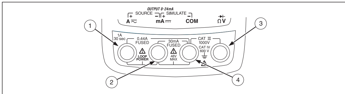
圖 2.輸入/輸出插口
