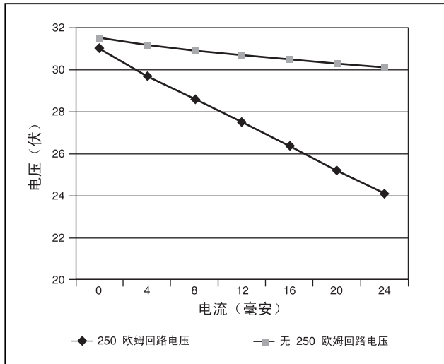
图 9。回路电压与电流
