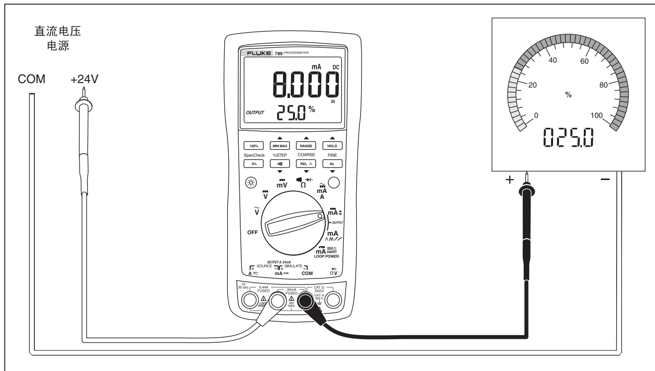
图 8。模拟变送器
