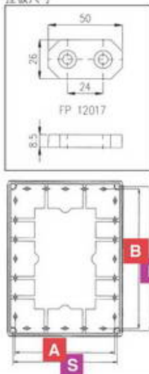
FP 12017 掛板尺寸
