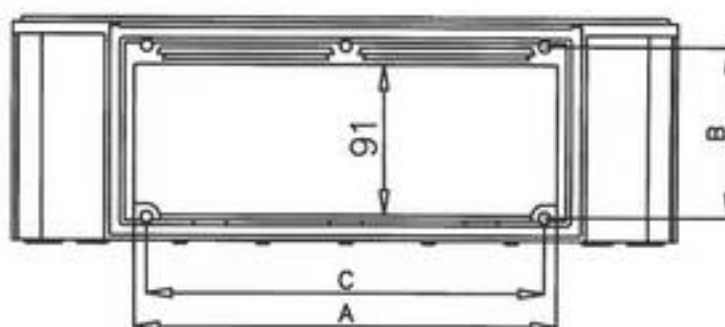
FIBOX EKI 法蘭開口 F2 及 F3 的外形圖及尺寸
