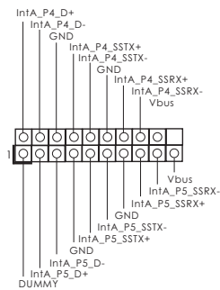
USB 3.0 扩展接头 (19 针 USB3_4_5) (见第 4 页第 9 项)
