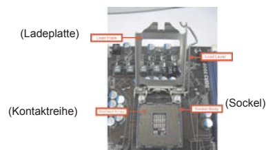
1155-Pin Sockel Übersicht
