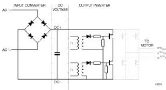
脉宽调制变频器电路原理图
