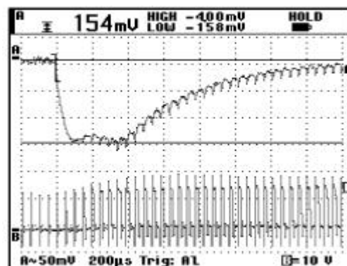
同时测量开关电源的输出和高频转换器的脉冲，可以得到反馈系统的响应
