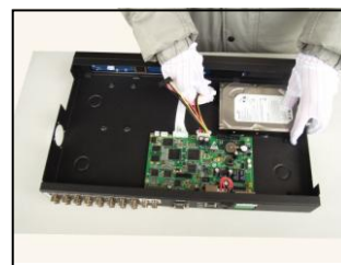
⑥连接硬盘电源线
