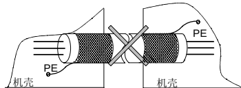
图 3-25 错误的屏蔽接地方法
