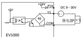
图 3-20 多功能输出端子接线方式 2
