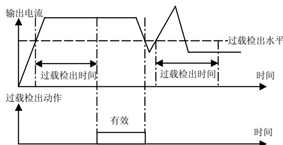
图 5-73 过载报警检出功能示意图
