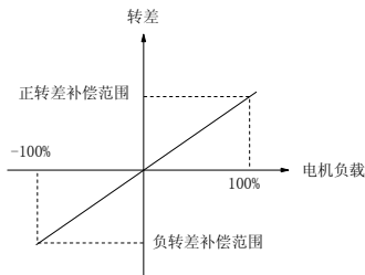
图 5-17 自动转差补偿
