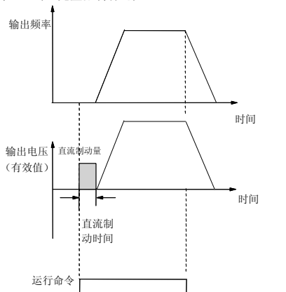
图 5-12 起动方式 1 说明
