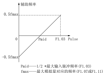
图 5-61 PULSE-0.5×F1.03 作为辅助频率给定通道
