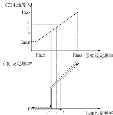
图 5-66 零频回差运行
