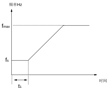
图 5-11 起动频率与起动时间示意图
