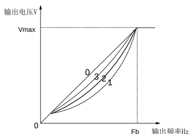
图 5-5 降转矩曲线
