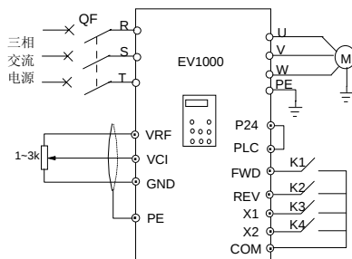
图 5-57 两地控制硬件接线图
