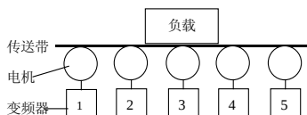
图 5-64 下垂控制示意图
