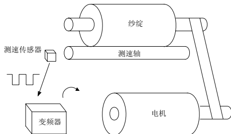
图 5-67 定长停机功能的应用
