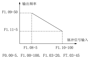
图 5-10 脉冲信号输入实例参数设置
