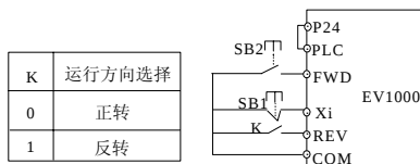
图 5-44 三线式运转模式 2
