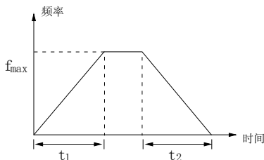
图 5-13 直线加减速
