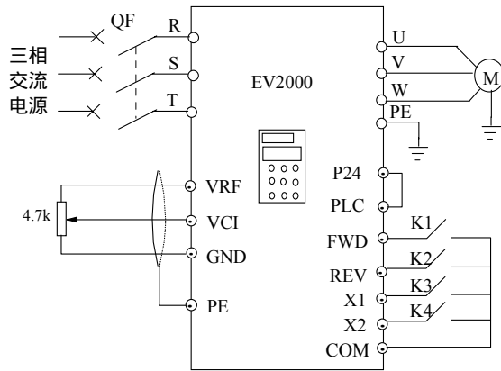
图5-58 两地控制硬件接线图
