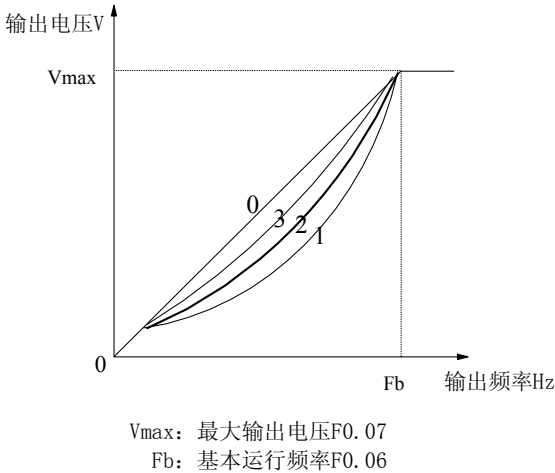
图5-5 降转矩曲线
