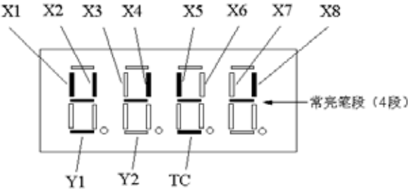
图5 - 54 端子状态指示
