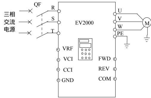
图3 - 7 主回路简单配线图
