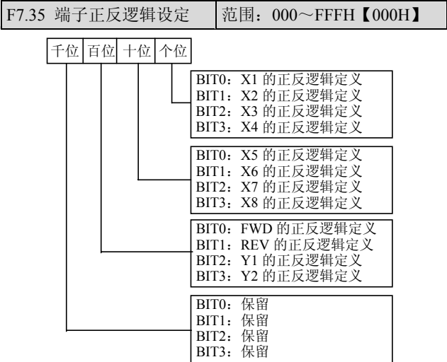
图5 - 51 端子正反逻辑设定
