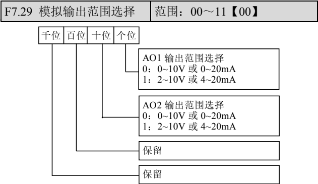
图5 - 49 模拟输出偏置设定
