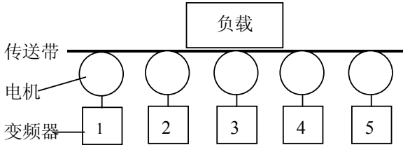
图5 - 65 下垂控制示意图
