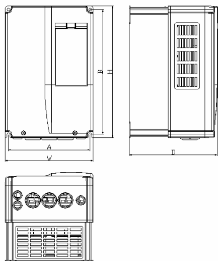
图a EV2000-4T0055G/0075P ~ EV2000-4T0150G/0185P
