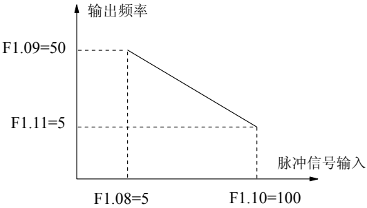
图5 - 10 脉冲信号输入实例参数设置
