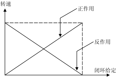
图5 - 33 闭环调节特性示意图
