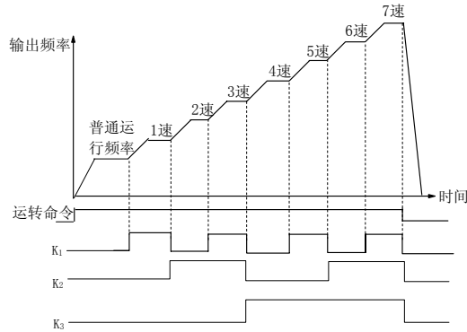
图5-39 多段速度运行示意图
