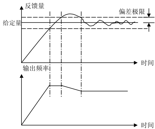
图5-35 偏差极限示意图
