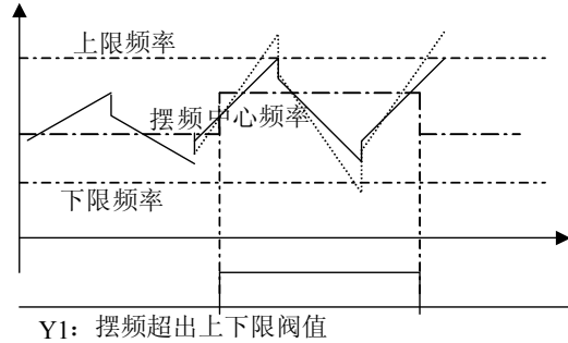
图5 - 46 摆频幅度限制
