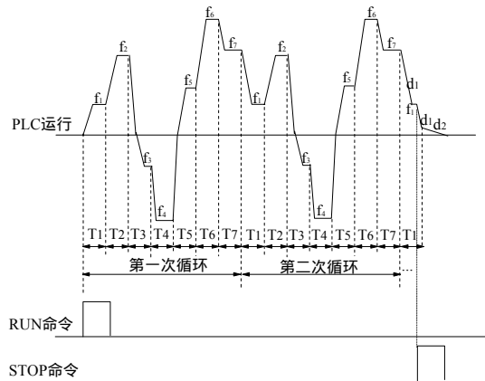
图5-25 PLC连续循环方式
