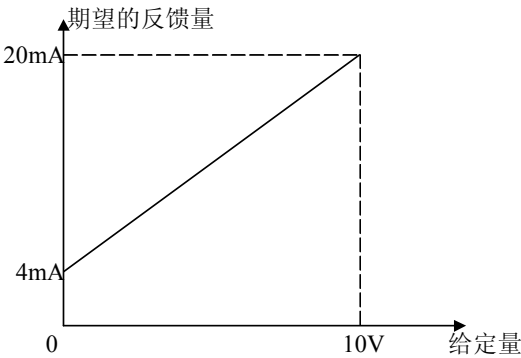
图5 - 32 给定量和期望反馈量
