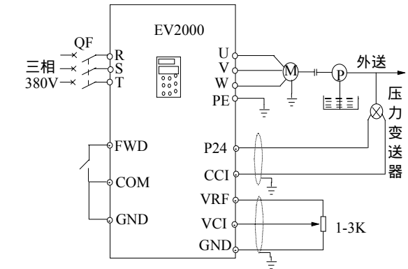
图5 - 29 内置PI模拟反馈控制系统示意图
