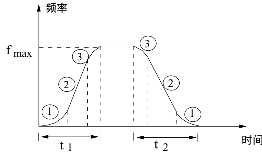
图5-15 S曲线加减速
