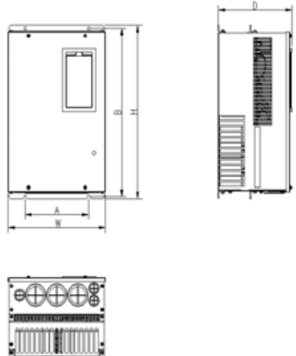
图b EV2000-4T0185G1/0220P1 ~ EV2000-4T0220G1/0300P1
