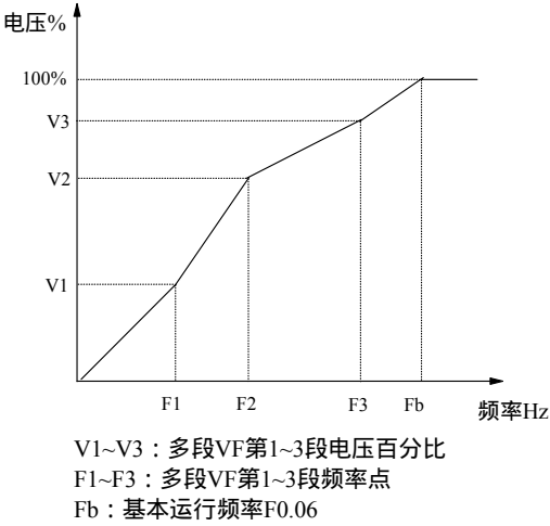
图5-6 用户设定V/F曲线一般形式
