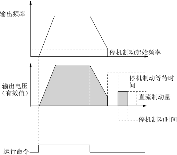
图5 - 16 减速停车+直流制动示意图
