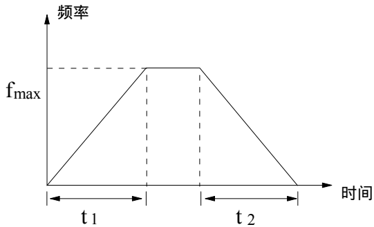
图5-14 直线加减速
