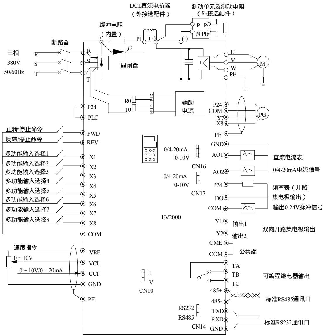
图3 - 11 基本配线图 3
