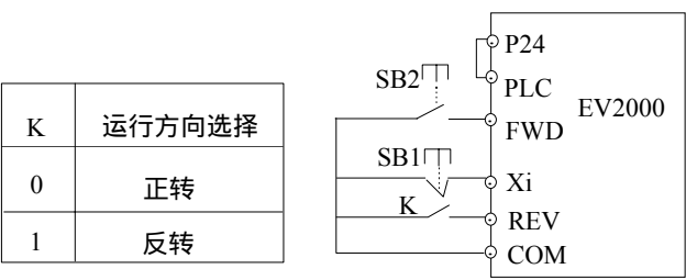
图5 - 45 三线式运转模式2
