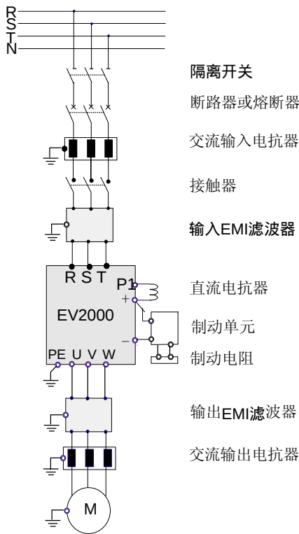
图3 - 8 变频器与选配件的连接
