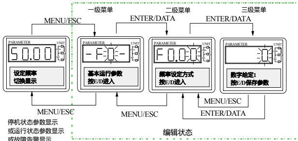
图4 - 6 操作面板的编程显示状态
