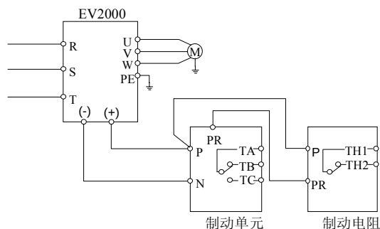
图2 - 10 变频器与制动组件连线图
