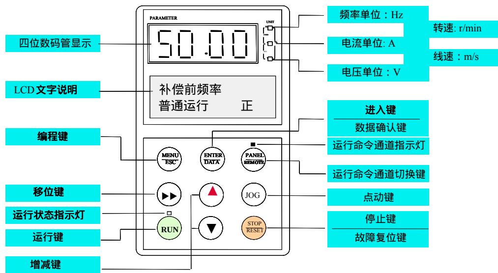
图4 - 2 操作面板示意图
