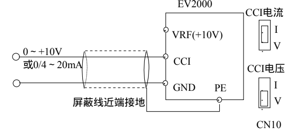
图3 - 15 CCI端子配线图
