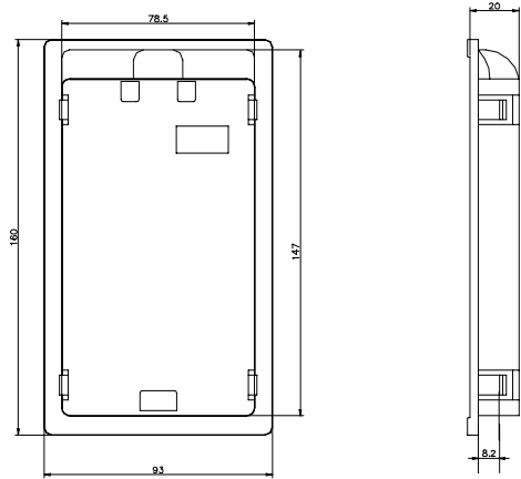
图b 安装盒
