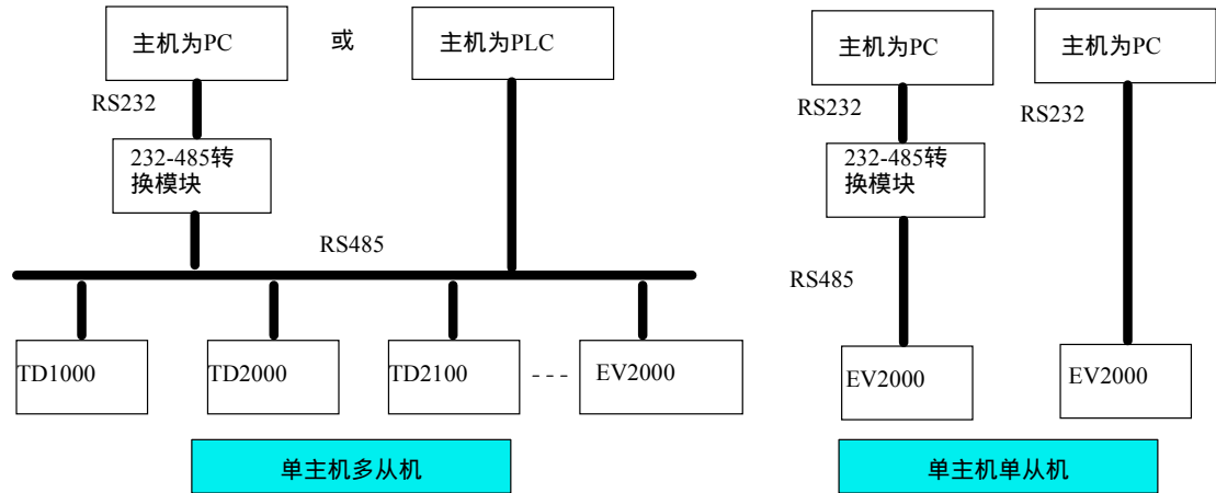
附图6 变频器组网方式示意图
