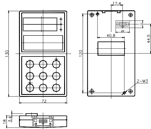
图a 操作面板
