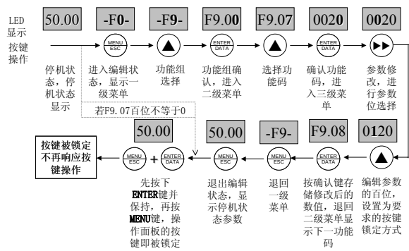
图4-14 操作面板按键锁定的操作示例
