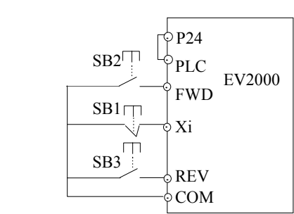
图5 - 44 三线式运转模式1
