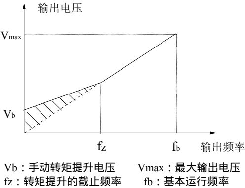
图5-3 转矩提升（提升量为阴影部分）
