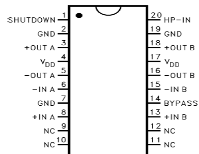
TSSOP-20
