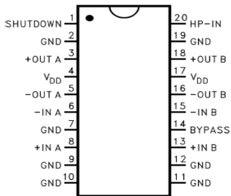
TSSOP-20
