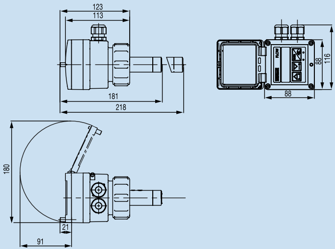
尺寸（包括接头）[mm]
