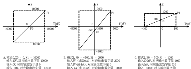
图 3-3 输入通道特性更改举例
