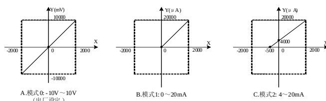
图 3-5 不更改各输出通道的 X0、X1 值, 各种模式对应通道特性
