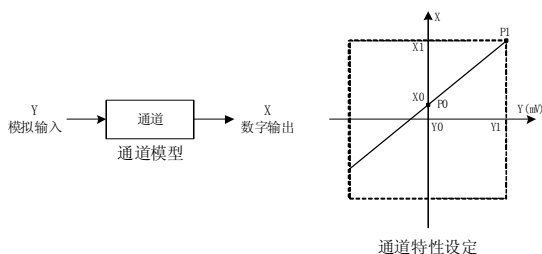
图 3-1 EC20-4AM 的输入通道特性示意图
