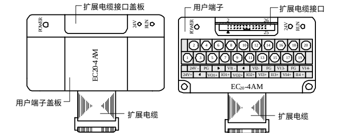
图 1-1 模块接口外观图 图 1-2 模块接口端子图
