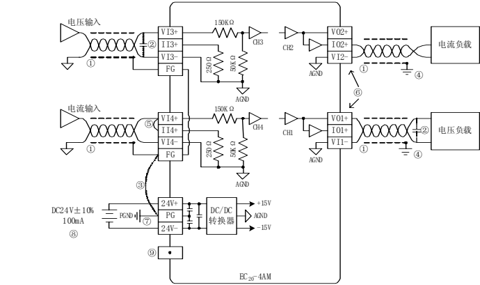
图 1-4 用户端子布线示意图
