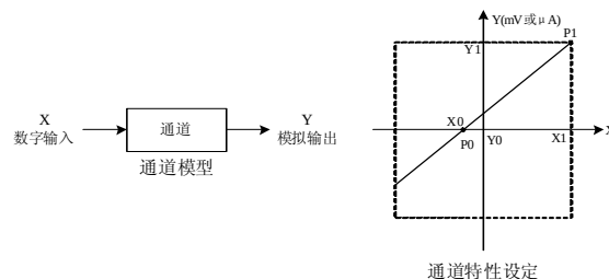
图 3-4 EC20-4AM 的输出通道特性示意图
