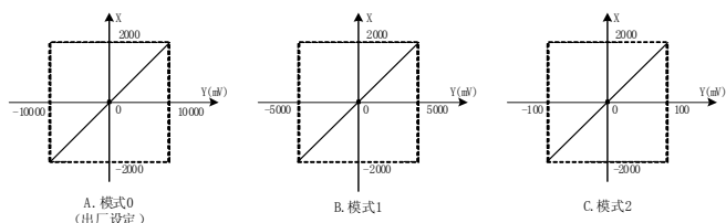
图 3-2 不更改各输入通道的 X0、X1 值, 各种模式对应通道特性
