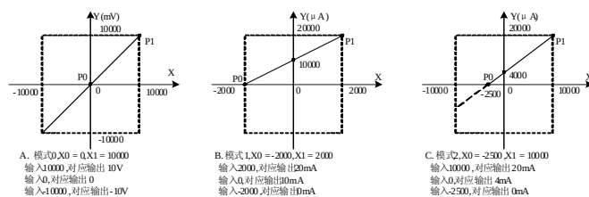
图 3-6 输出通道特性更改举例
