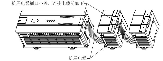
图 1-3 与主模块的连接示意图
