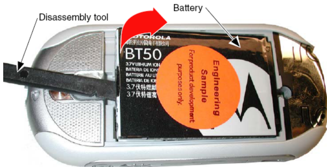
图8. 拆卸电池
