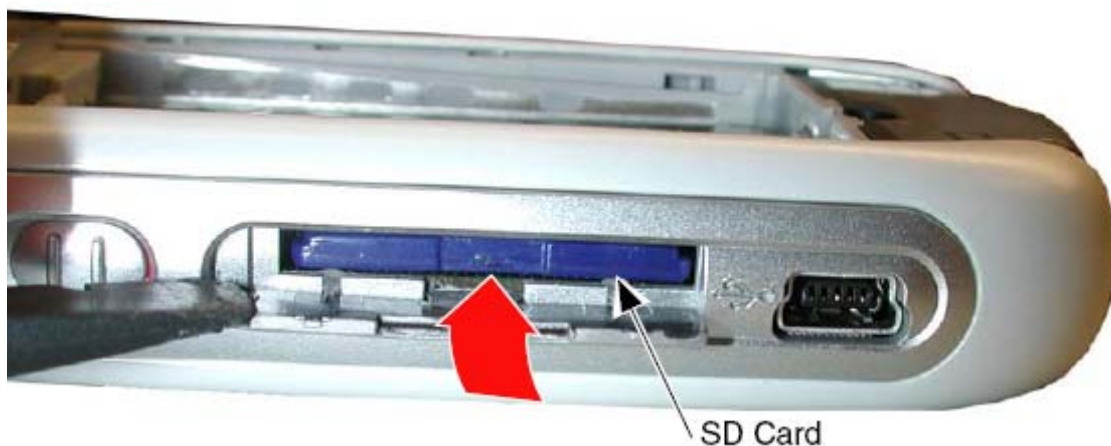
图5. 拆卸存储卡
