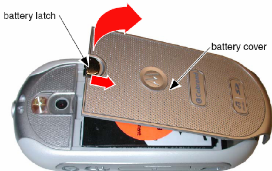
图7. 拆卸电池门
