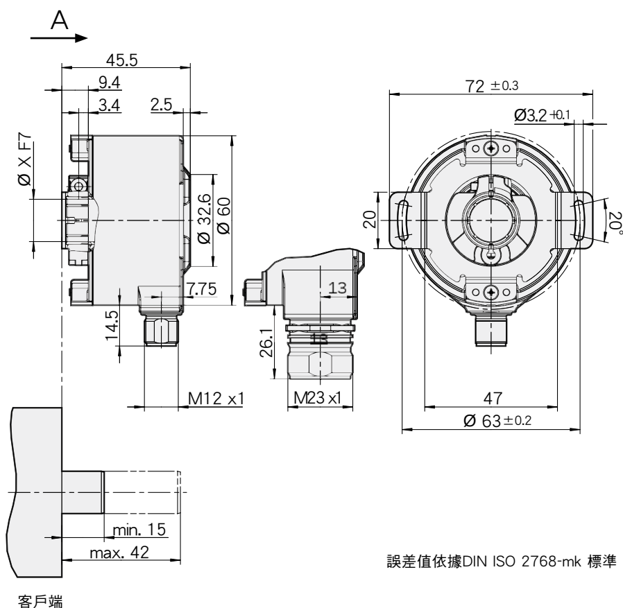
尺寸圖-半中空 - M12與M23插座
