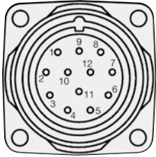
M23 插座腳位圖
