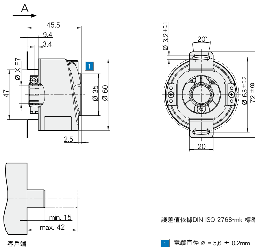
尺寸圖-半中空軸 - 電纜出線
