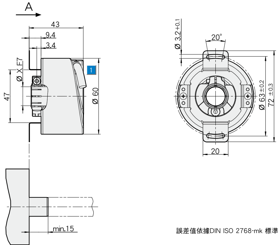
尺寸圖-金屬中空軸-電纜出線
