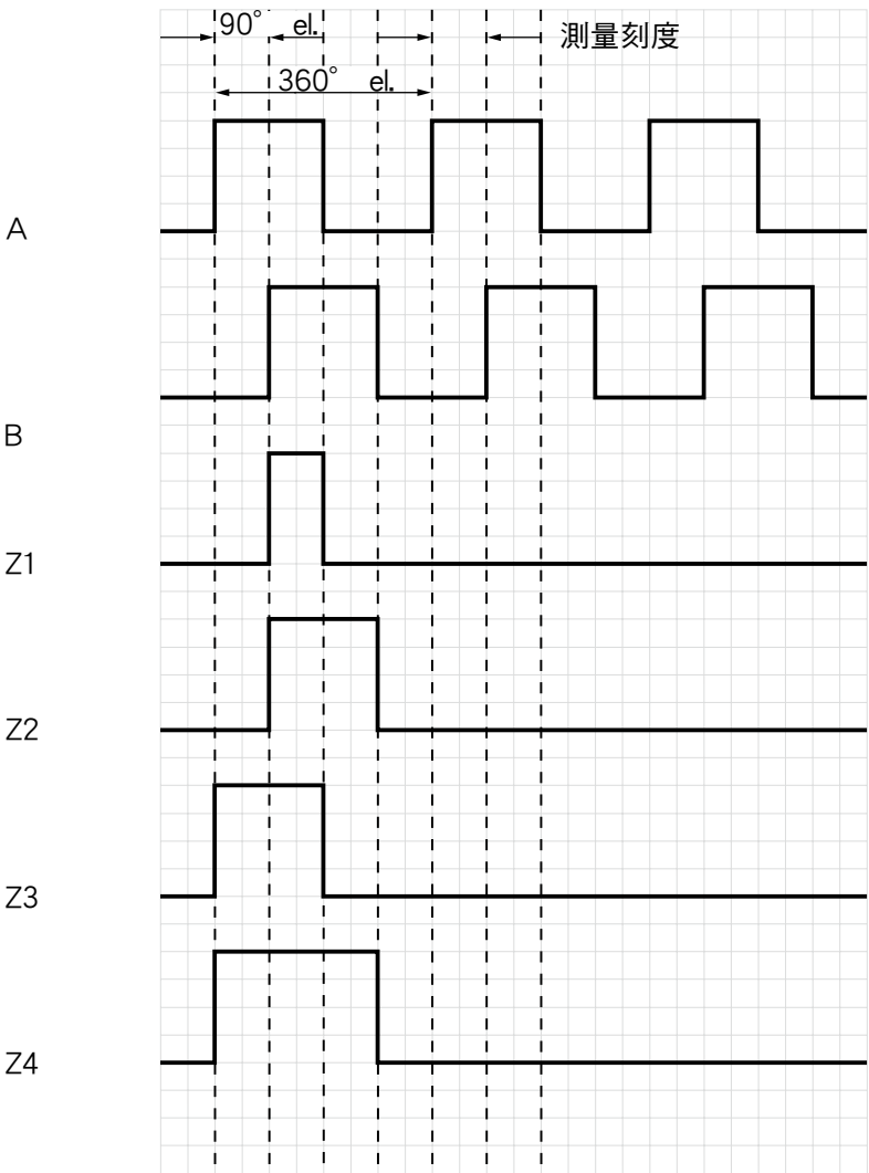
尺寸圖A的順時針方向
