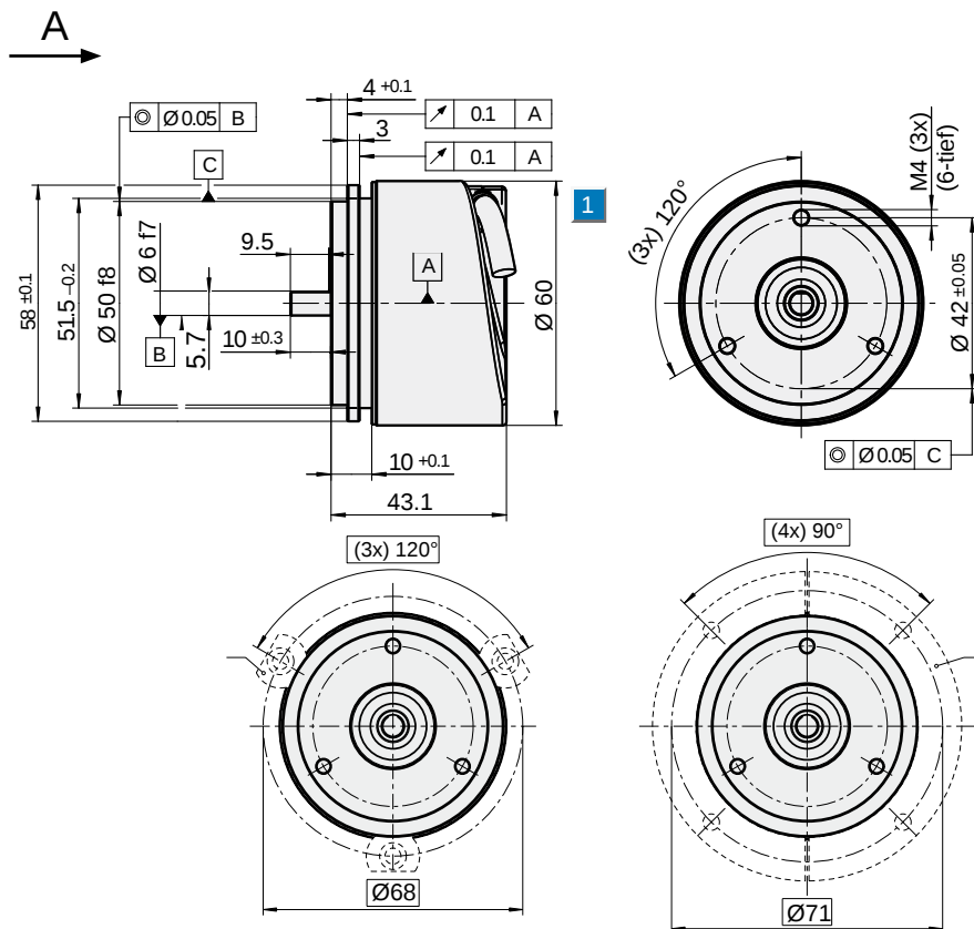
尺寸圖 - 電纜出線
