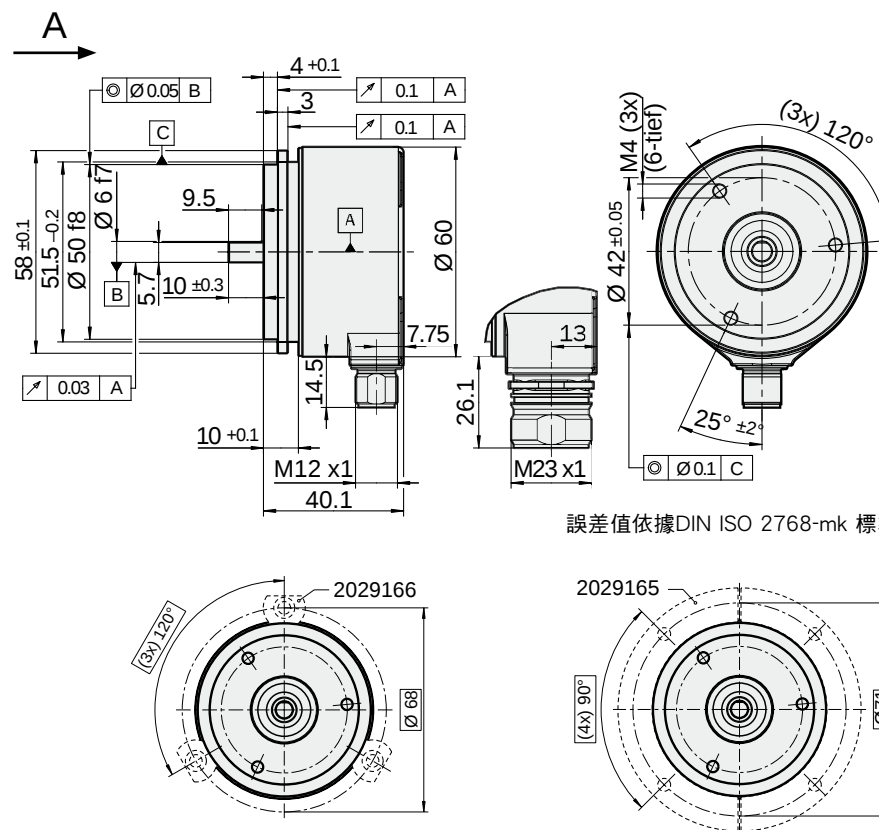
尺寸圖伺服凸緣 - M12與M23插座
