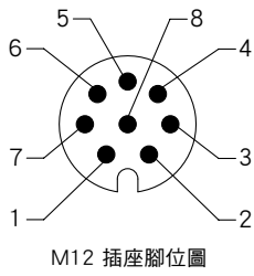
M12 插座腳位圖
