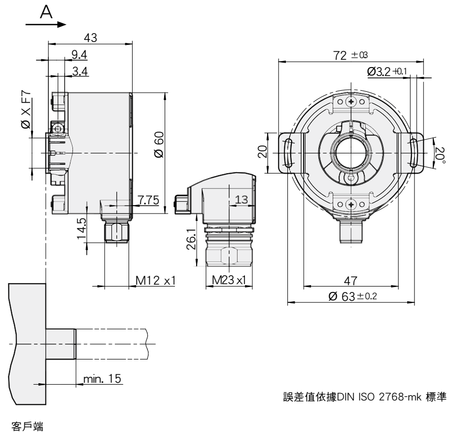
尺寸圖-金屬中空軸 - M12與M23插座
