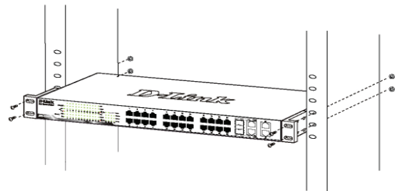
Abbildung 3: Switch im Standardrack installieren
