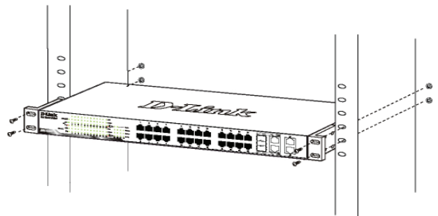
Gambar 3. Memasang switch ke rak dengan ukuran standar
