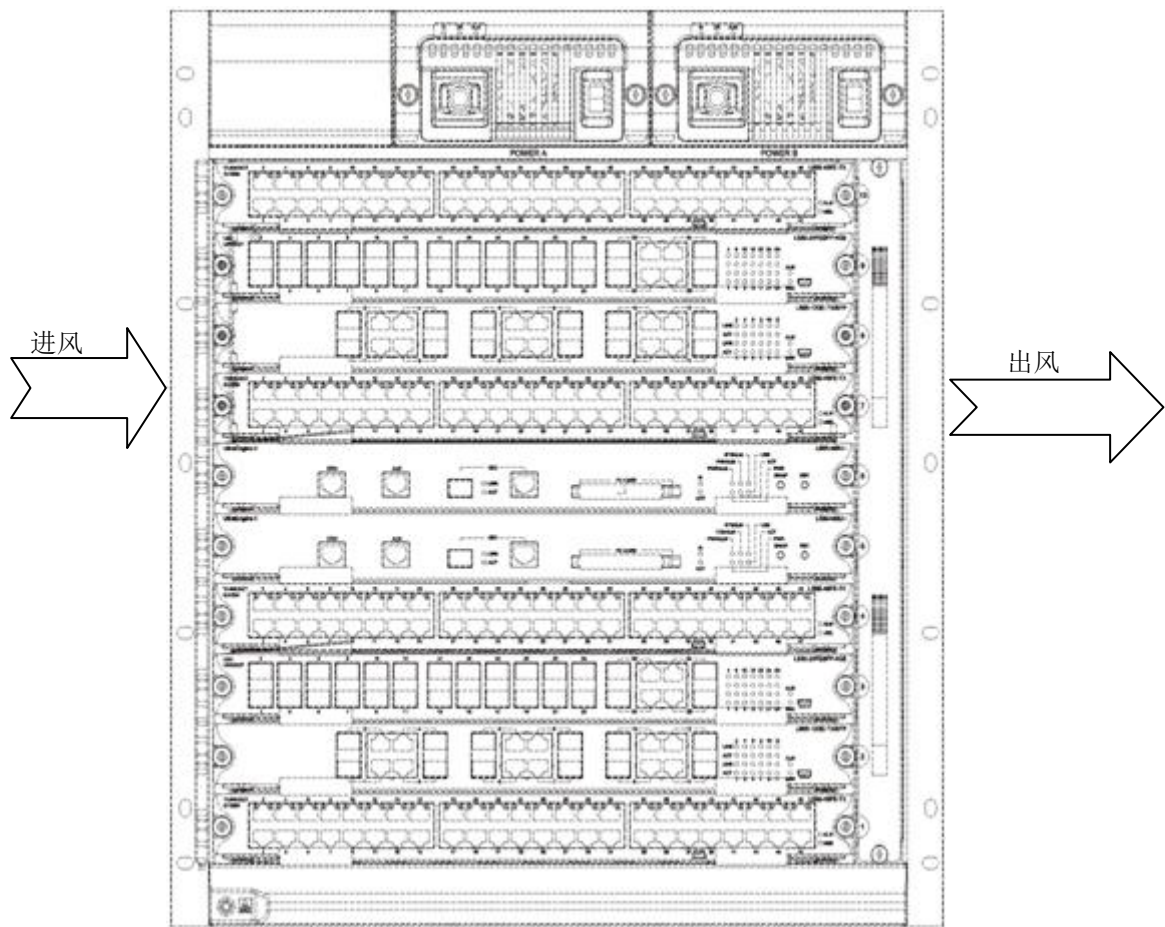
图 1-10 DES-8500 通风散热对流方案图
