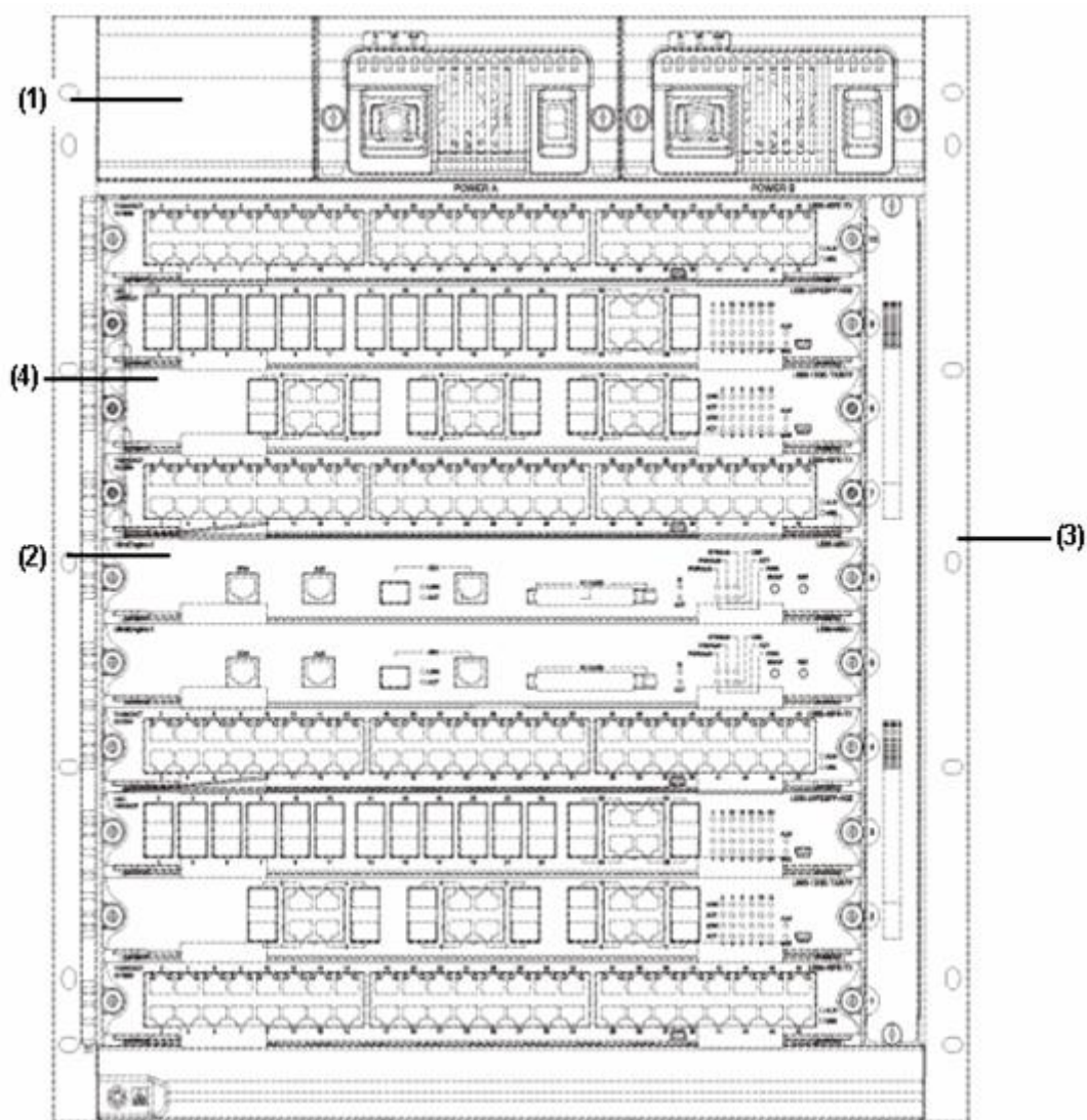
图 1-3 DES-8510 外观图
