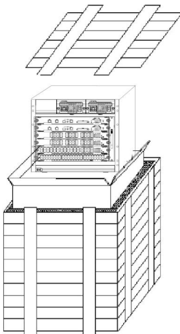
图 5-1 设备包装图
