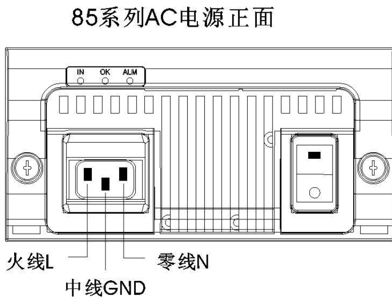
图 3-2 交流电源连接示意图
