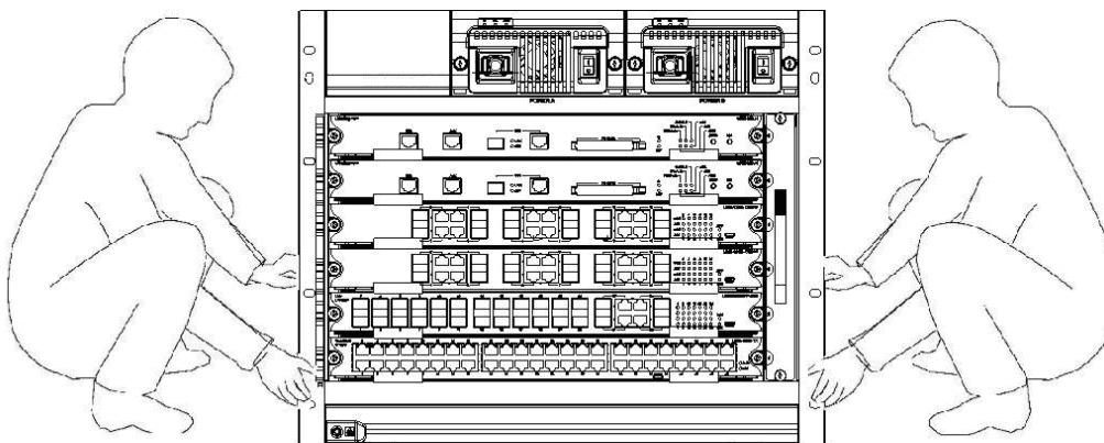
图 2-1 正确搬运 DES-8500 示意图
