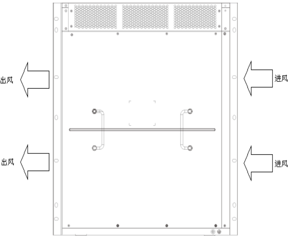
图 2-2 DES-8500 通风方式
