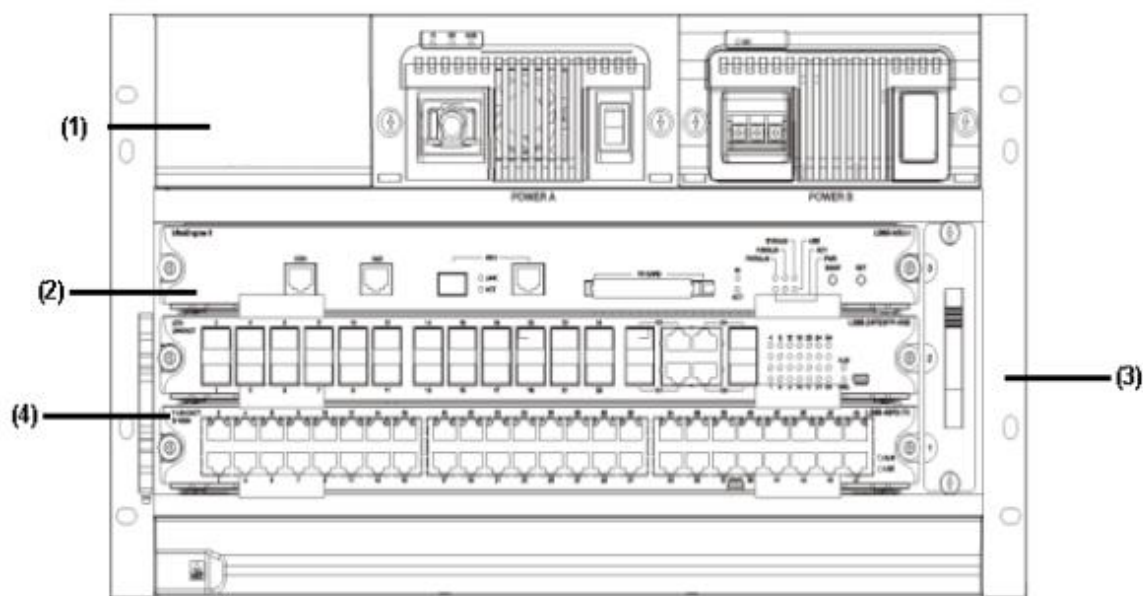
图 1-1 DES-8503 外观图
