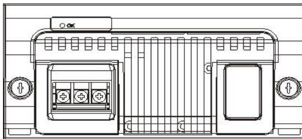
图 1-8 直流电源前面板
