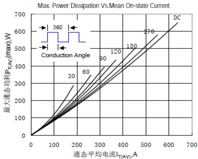
Fig.5 最大功耗与平均电流关系曲线
