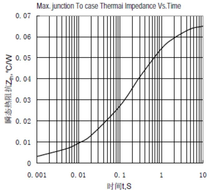
Fig.2 结至管壳瞬态热阻抗曲线
