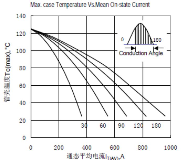
Fig.4 管壳温度与通态平均电流关系曲线
