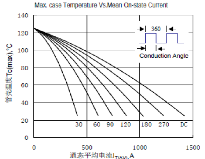
Fig.6 管壳温度与通态平均电流关系曲线
