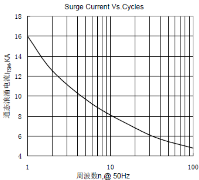
Fig.7 通态浪涌电流与周波数的关系曲线
