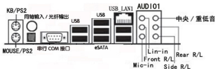
此图为断剑 C.A770 Ver1.7A 主板后面板
