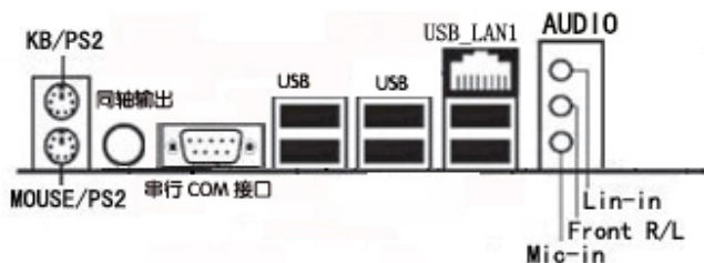
此图为断剑 C.A770T Ver1.7A 主板后面板
