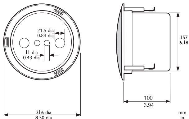
带 LBC 3081/02 防火罩组件的 LBC 3086/41 扬声器尺寸 (单位: 毫米 [英寸])
