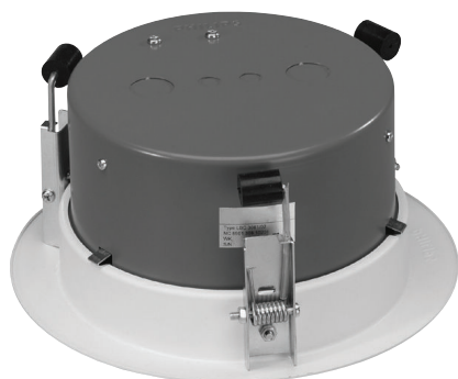
带 LBC 3081/02 防火罩组件的 LBC 3086/41 扬声器
