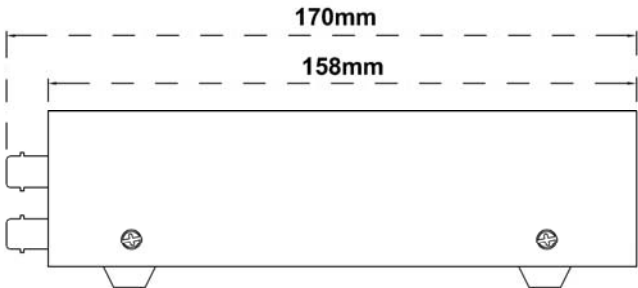
BN-8X16侧面示意图
