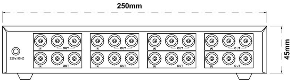
BN-8X16后面板示意图
