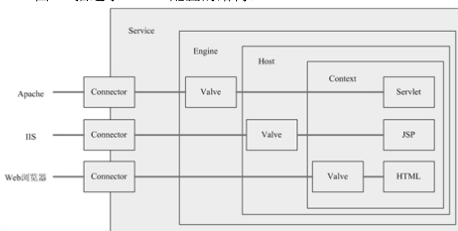
图 1-2 Tomcat 配置体系结构图
