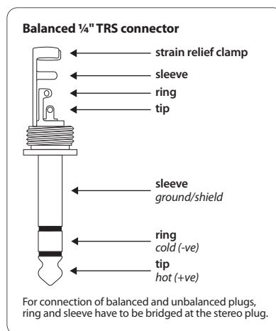
图 4.1 6.3 毫米立体声插头
