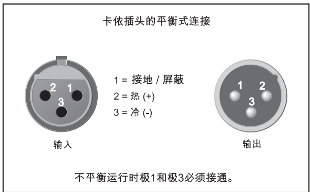
图 4. 2: XLR插头
