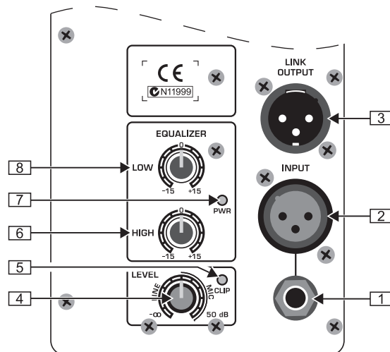
图 2.1: 操作元件和接口 (E1220A和E1520A)
