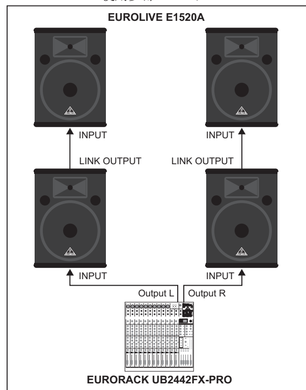
图 3.1: 多部E1220A/E1520A的接线通过LINK OUTPUT接口
