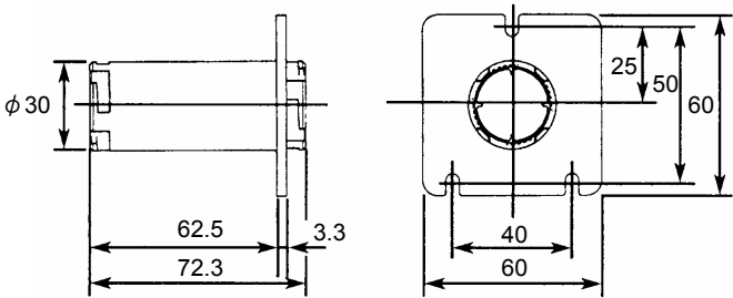
(3) 安装支架
