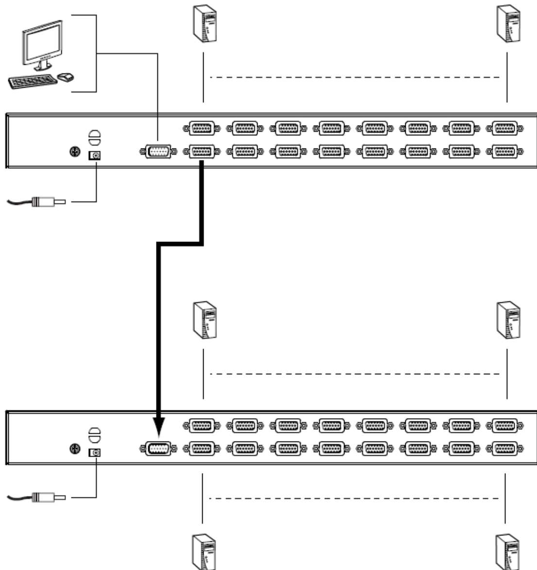
接続図(2段階構成)
